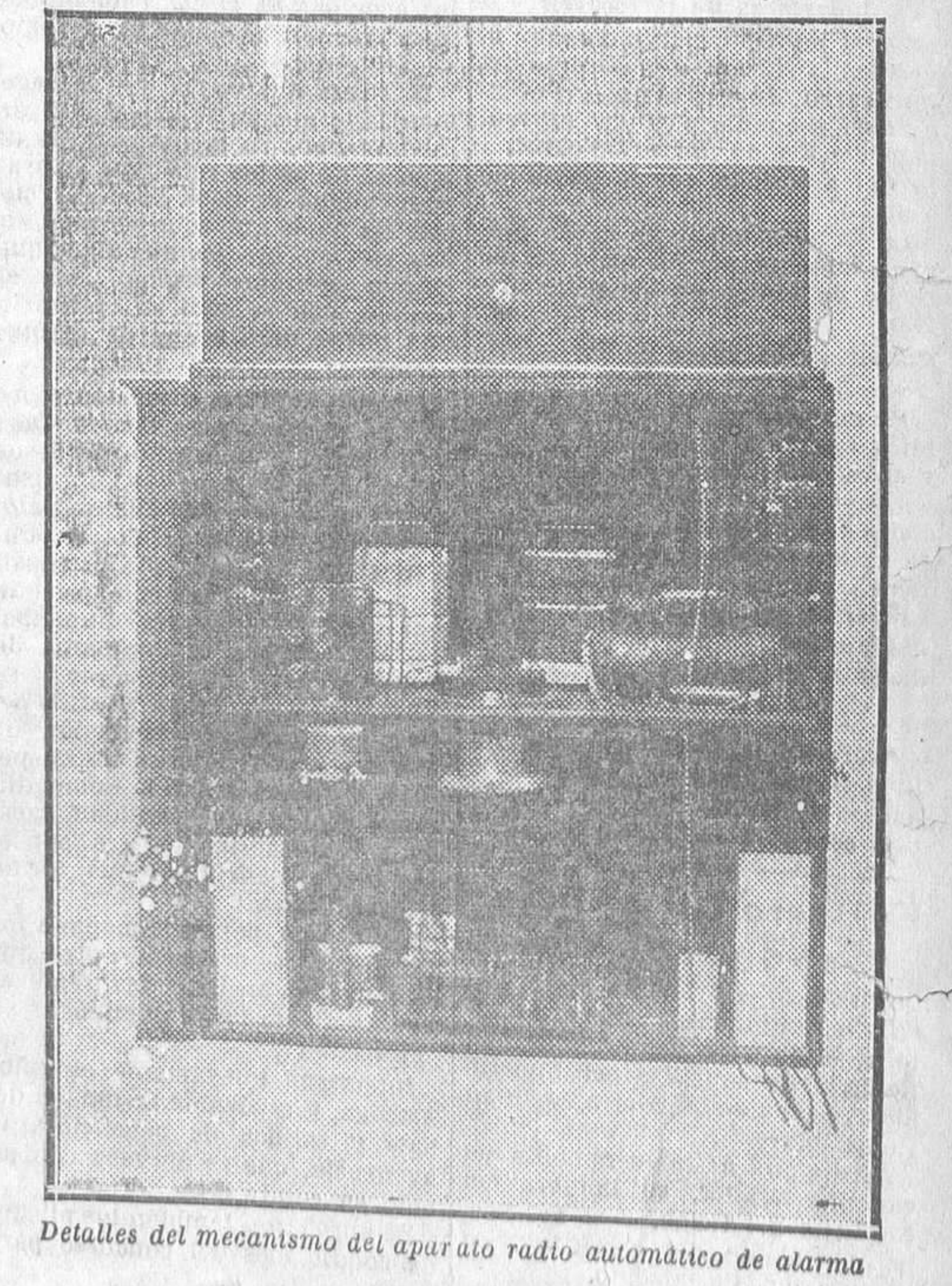
Detalles del mecanismo del aparato radio automático de alarma
