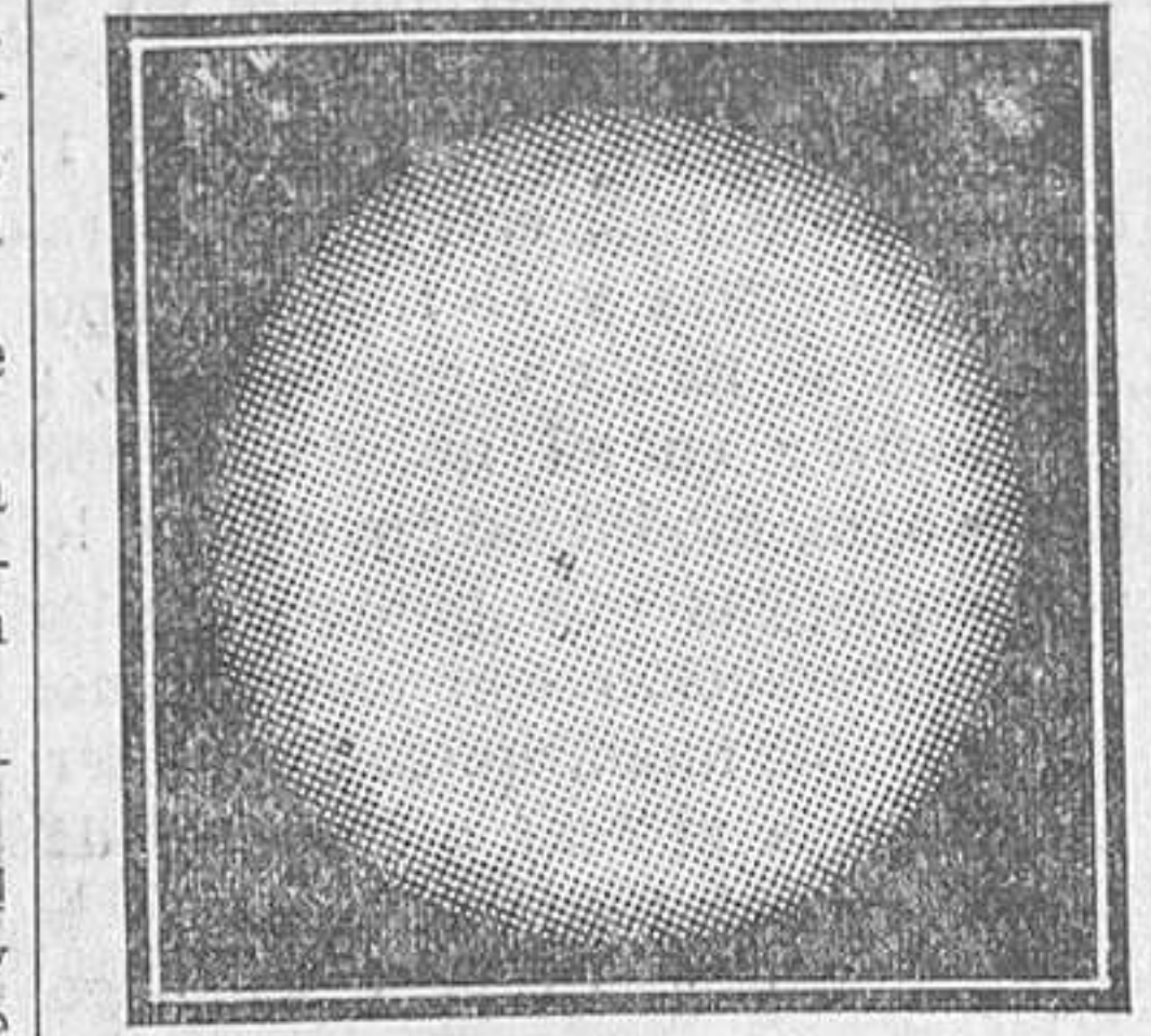
Paso de Mercurio ante el disco solar en 1907. Fotografía obtenida por el astrónomo Raurich, de Barcelona
