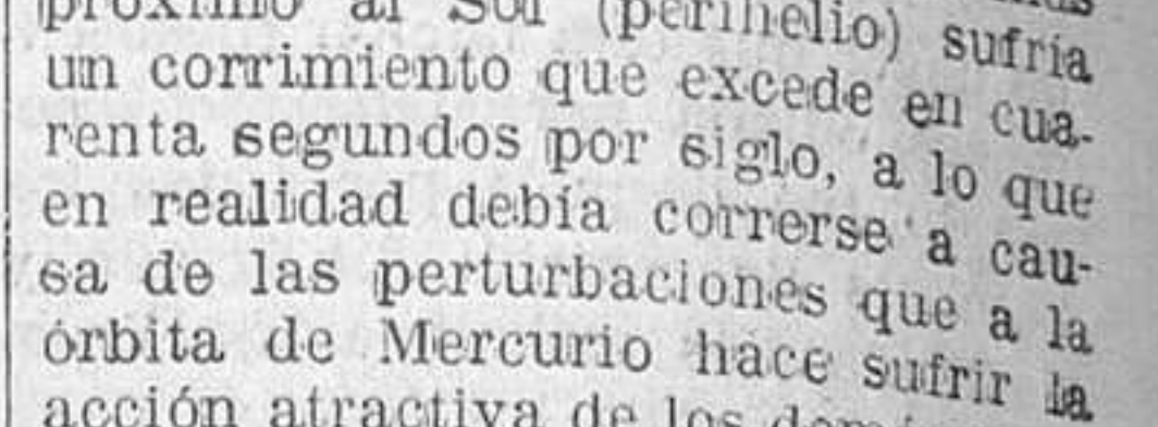
Orbita de Mercurio. El punto que dista unos 73° del punto N. del Sol hacia el Oeste.
