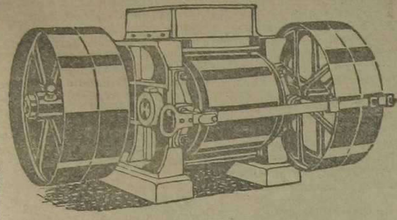
Laminador afinador, modelo F.A.-VIIIb
