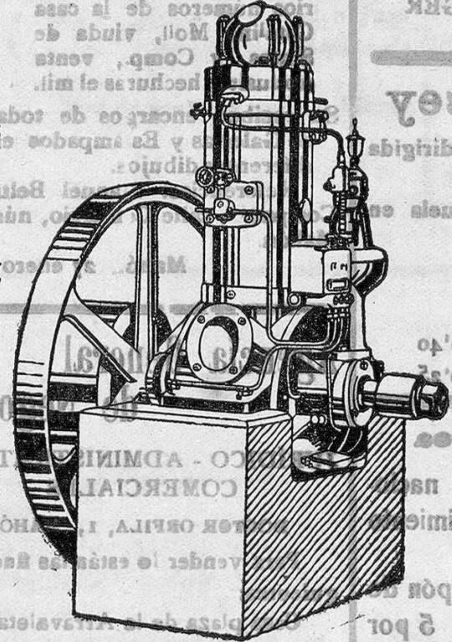
Motor para aceites pesados sin válvulas, sin magneto.
