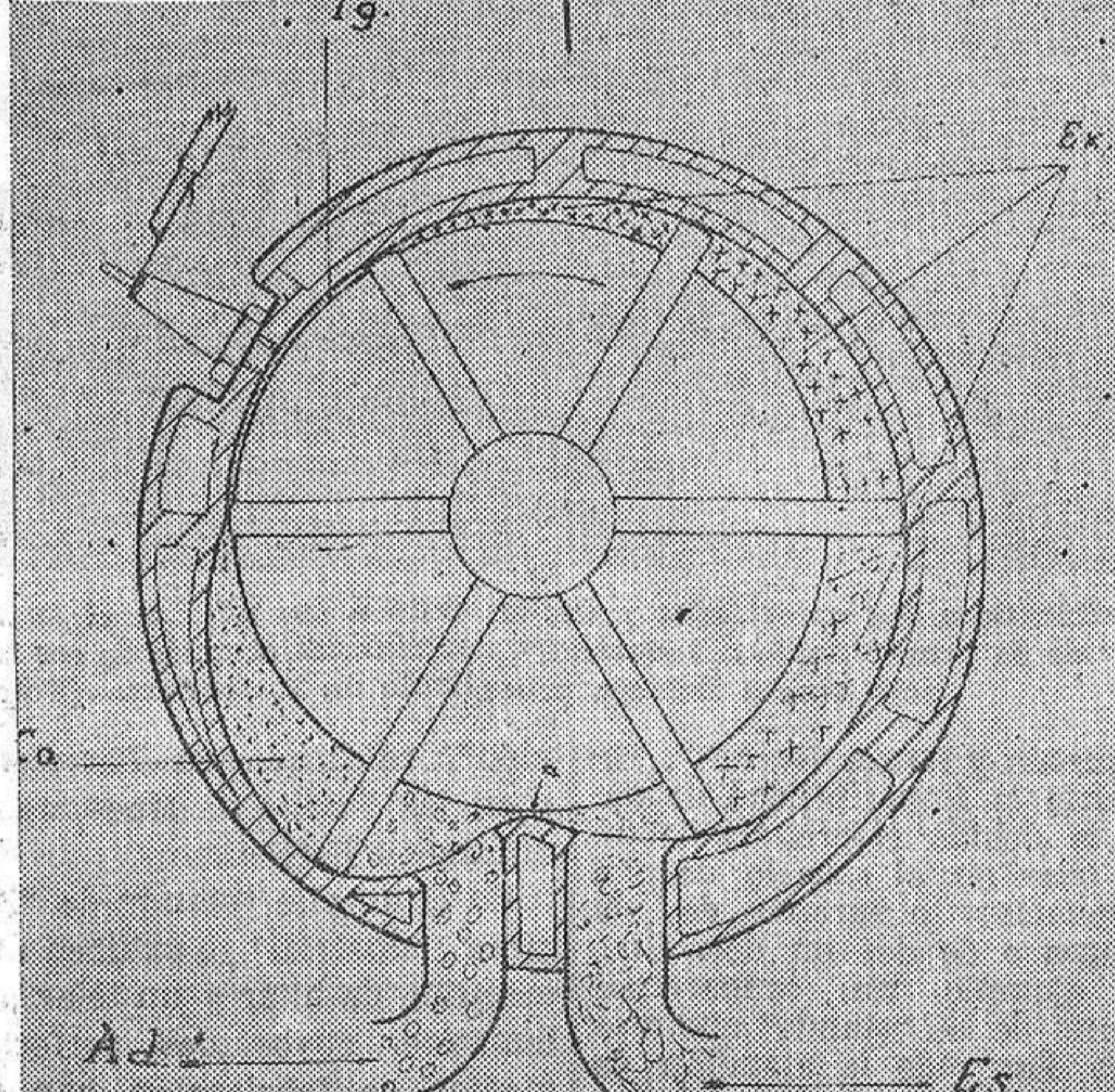
Ad.: Admisión.—Co.: Compresión.—Ig.: Ignición.—Ex.: Expansión.—Es.: Escape.
