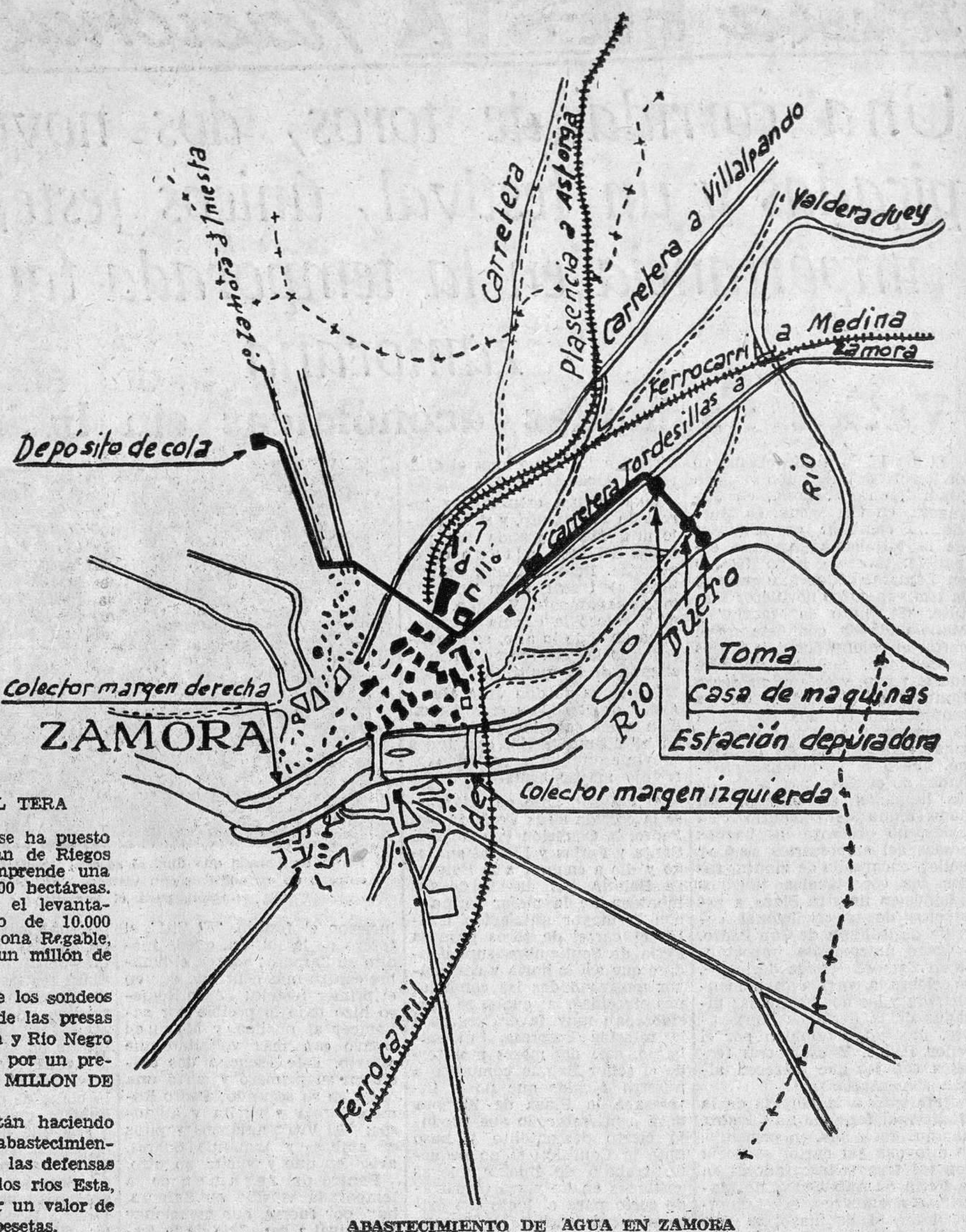
ABASTECIMIENTO DE AGUA EN ZAMORA
