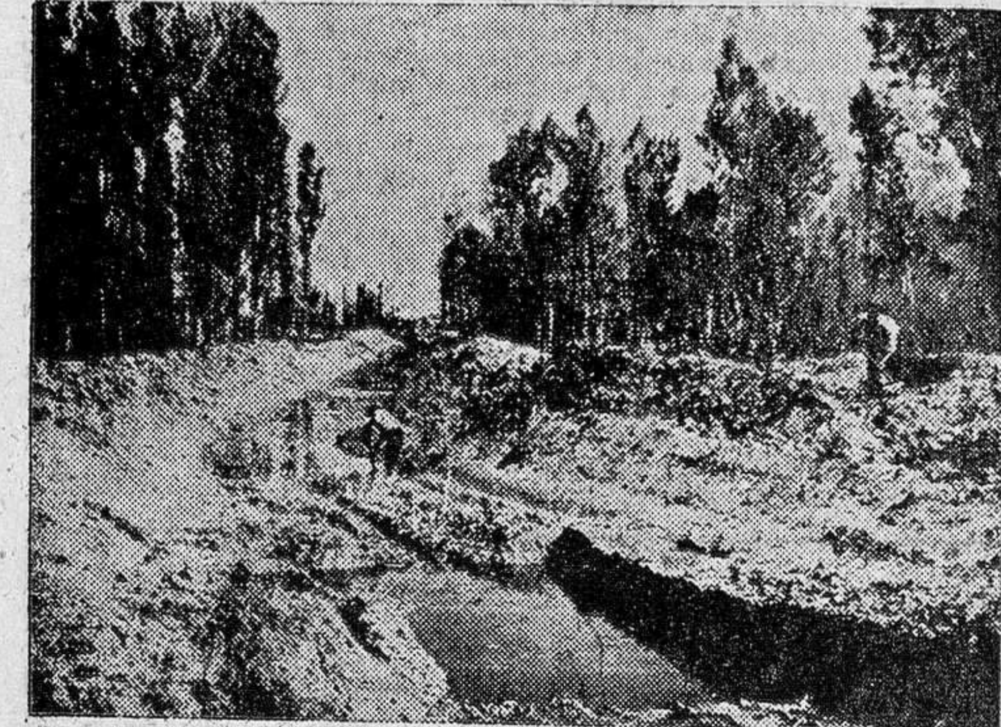
Obras de encauzamiento del arroyo de Valparaíso en Peleas de Abajo.
