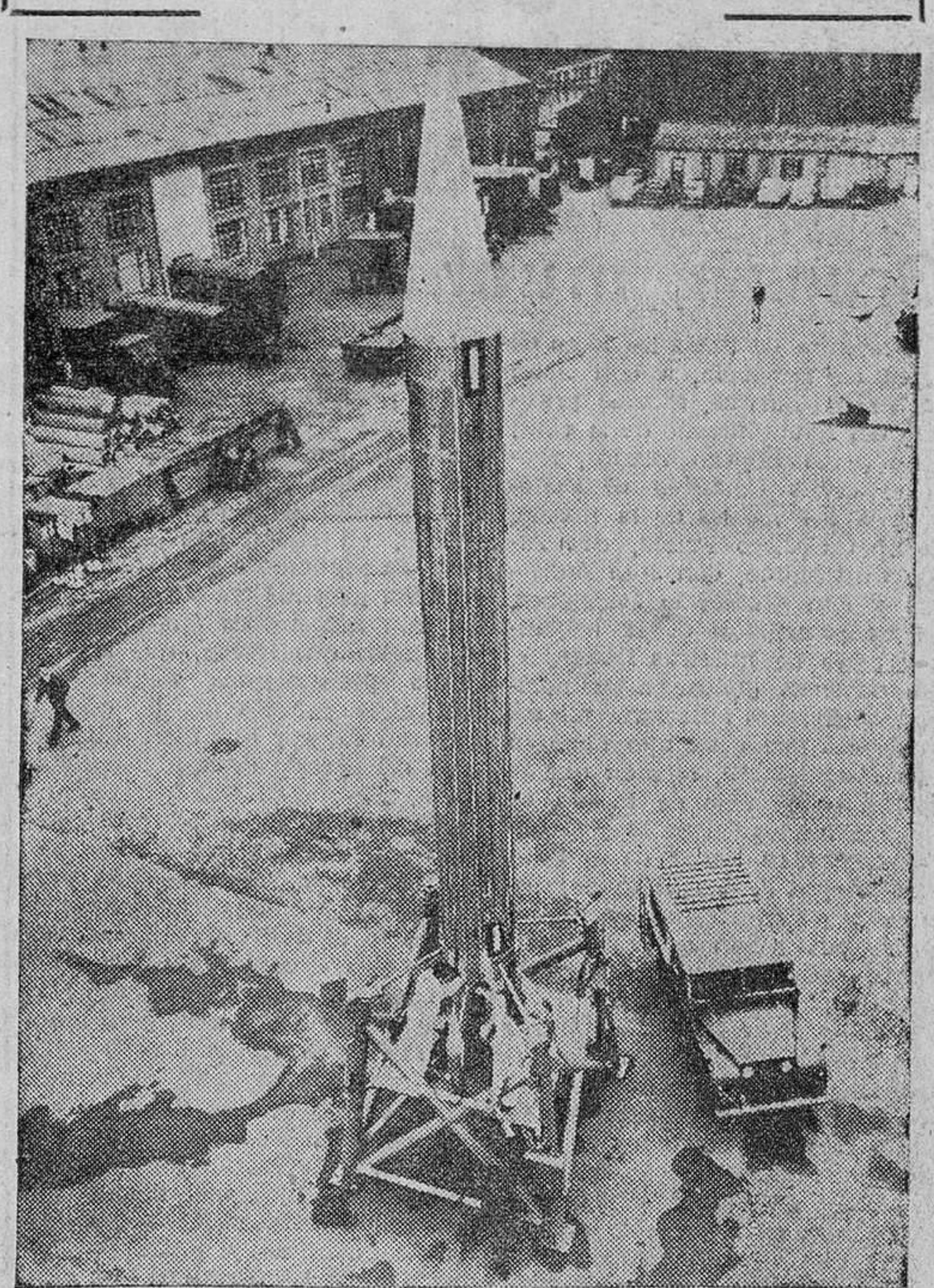
El proyectil americano «Black Knight», creado para investigaciones científicas, ha sido lanzado en Woomera (Australia) con el mayor de los éxitos. Tiene 35 pies de largo y tres de diámetro, y después de ser lanzado es controlado por un aparato que le hace moverse en la dirección apetecida. En la fotografía le podemos apreciar poco antes de su lanzamiento.
