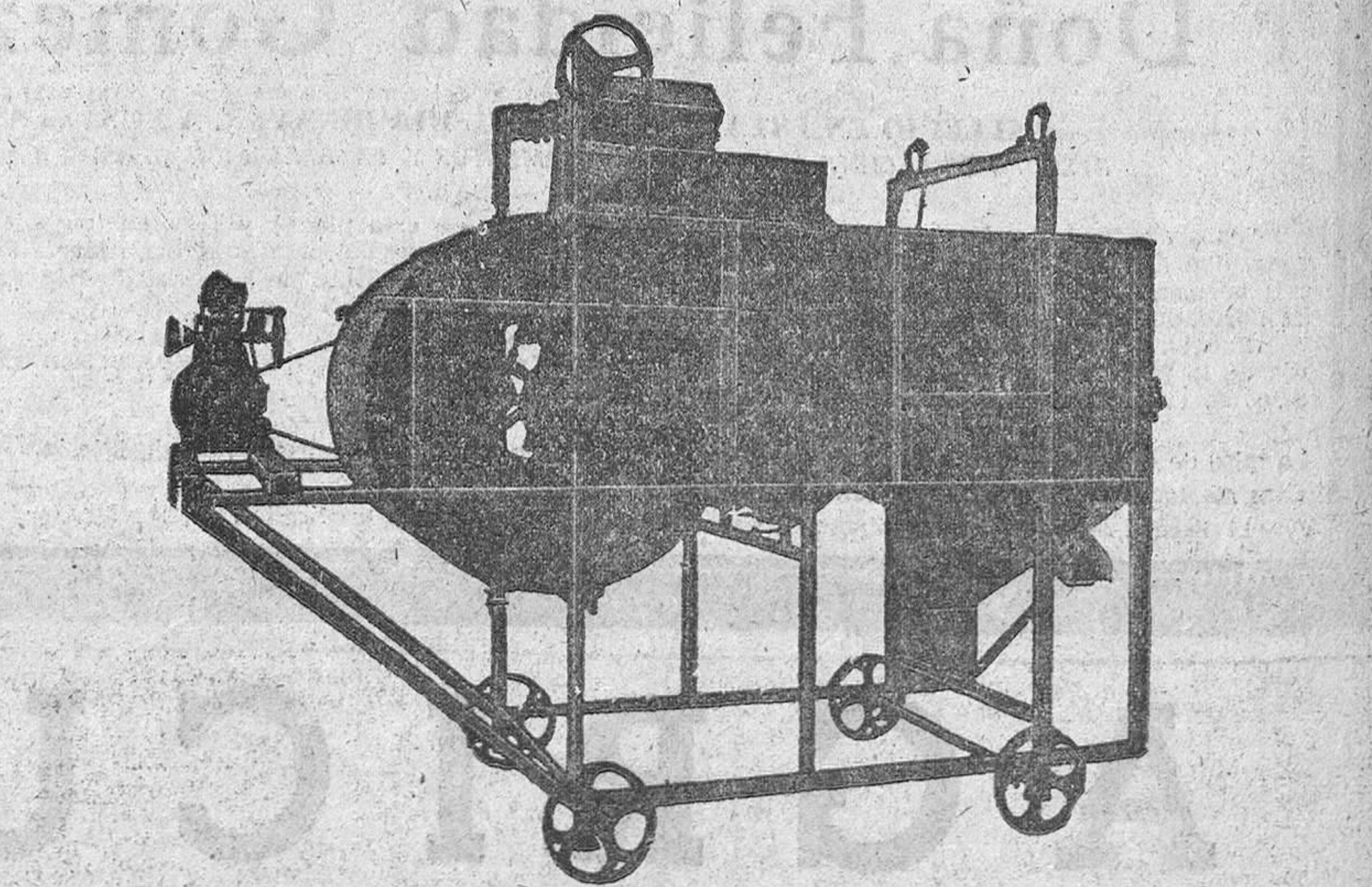
Aventadora Ensacadora Metálica de un metro y de 1,10 de luz, con zarandones y elevador de madera.
