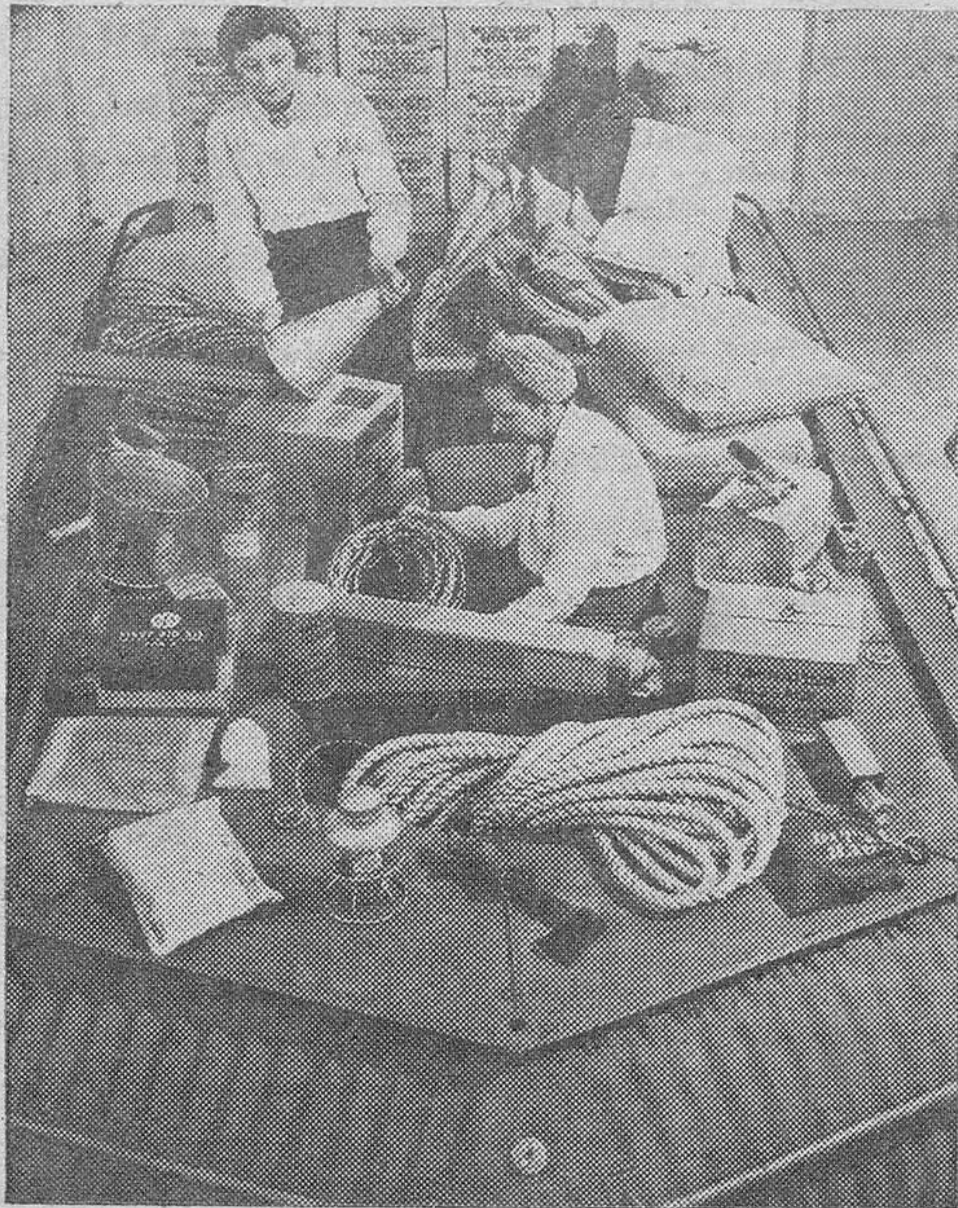
En la fábrica las obreras proceden a instalar las provisiones en una nueva balsa salvavidas para mercantes. Es totalmente metálica, contiene una estufa de carbón, una caparuzo de protección contra la lluvia y el viento, y viveros y agua para un mes.
