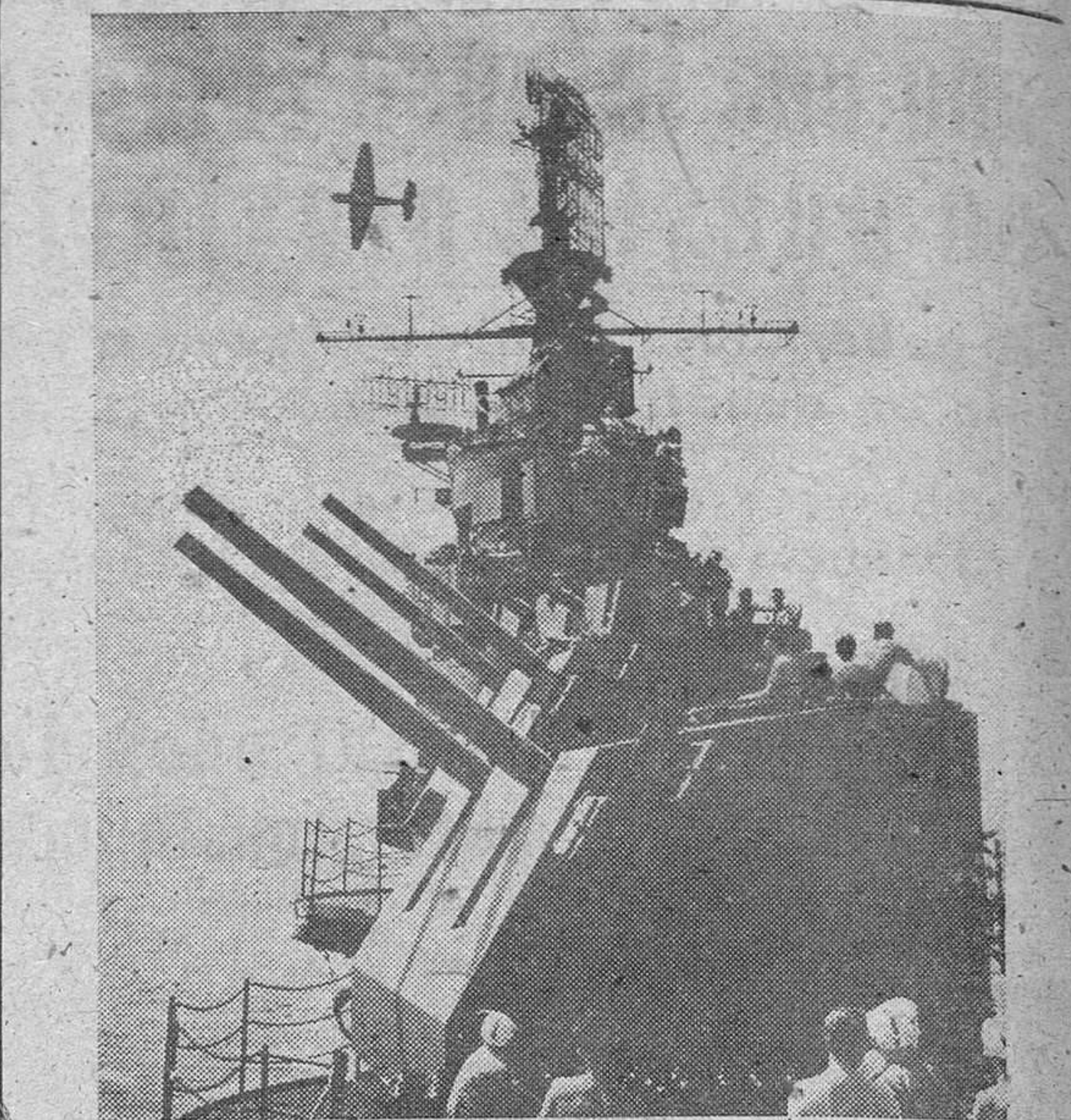
Un bombardero «Avenger» norteamericano, equipado con aparato Radar, pasa cerca de un portaaviones de 27.000 toneladas. Sobre el cielo puede verse dibujada la silueta de la antena del equipo Radar.
