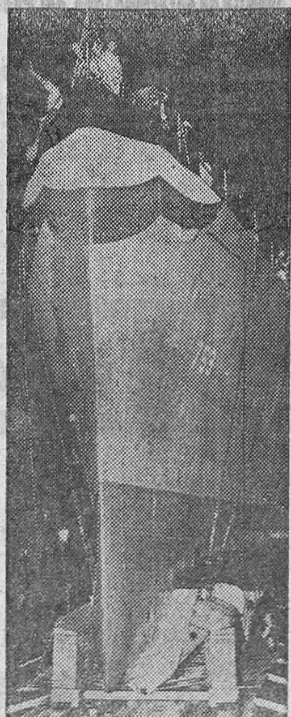
El superdestructor «Pierro» de 2.200 toneladas se desliza por la grada durante su botadura nocturna en un astillero de los EE. UU.
