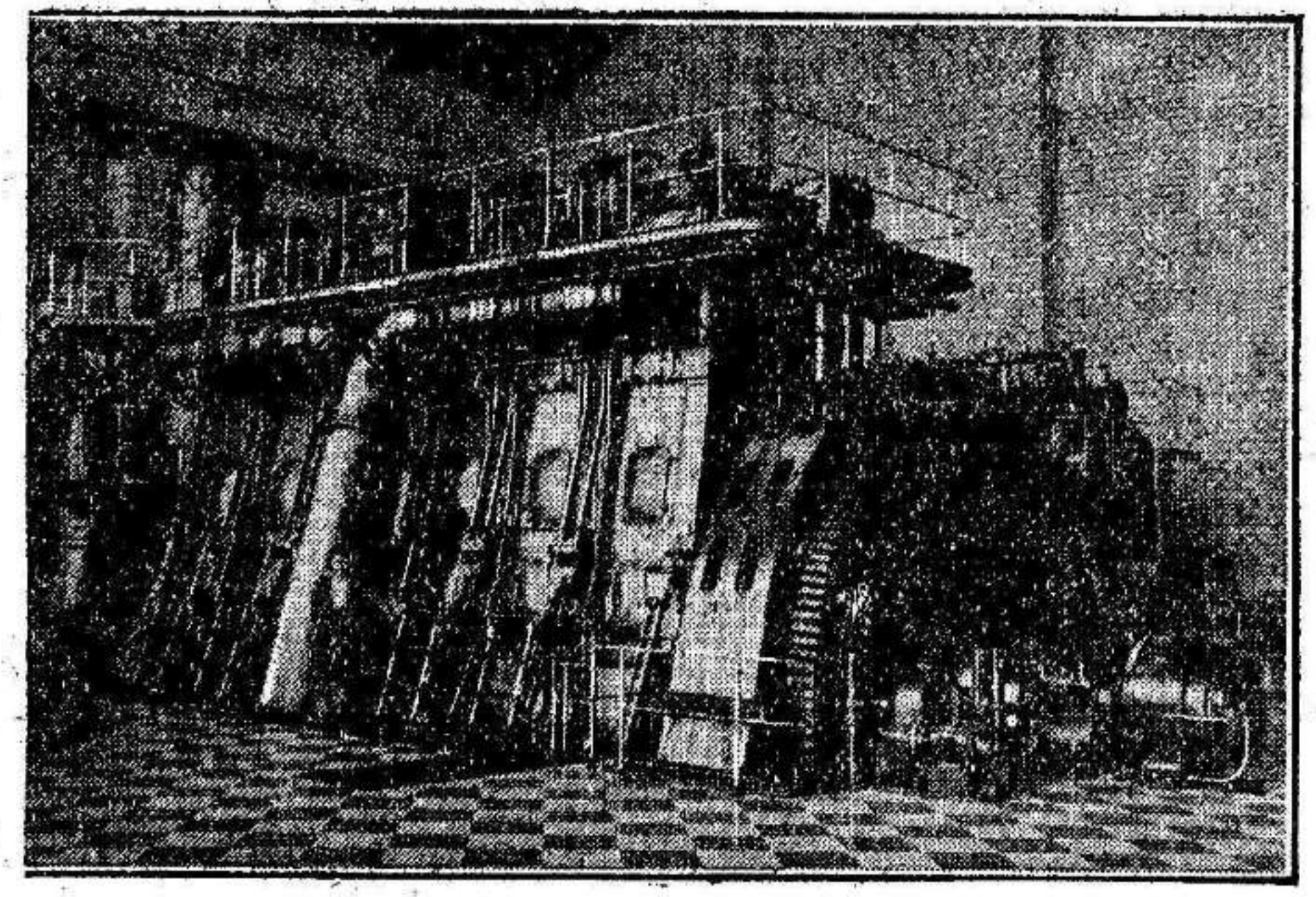
CENTRAL DE ALICANTE 2 MOTORES DIESEL DE 8.000 H. P.
