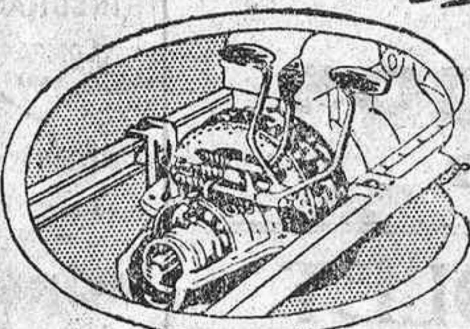
La transmisión planetaria FORD cuesta más fabricarse, pero es de más fácil funcionamiento por su sencillez y seguridad
