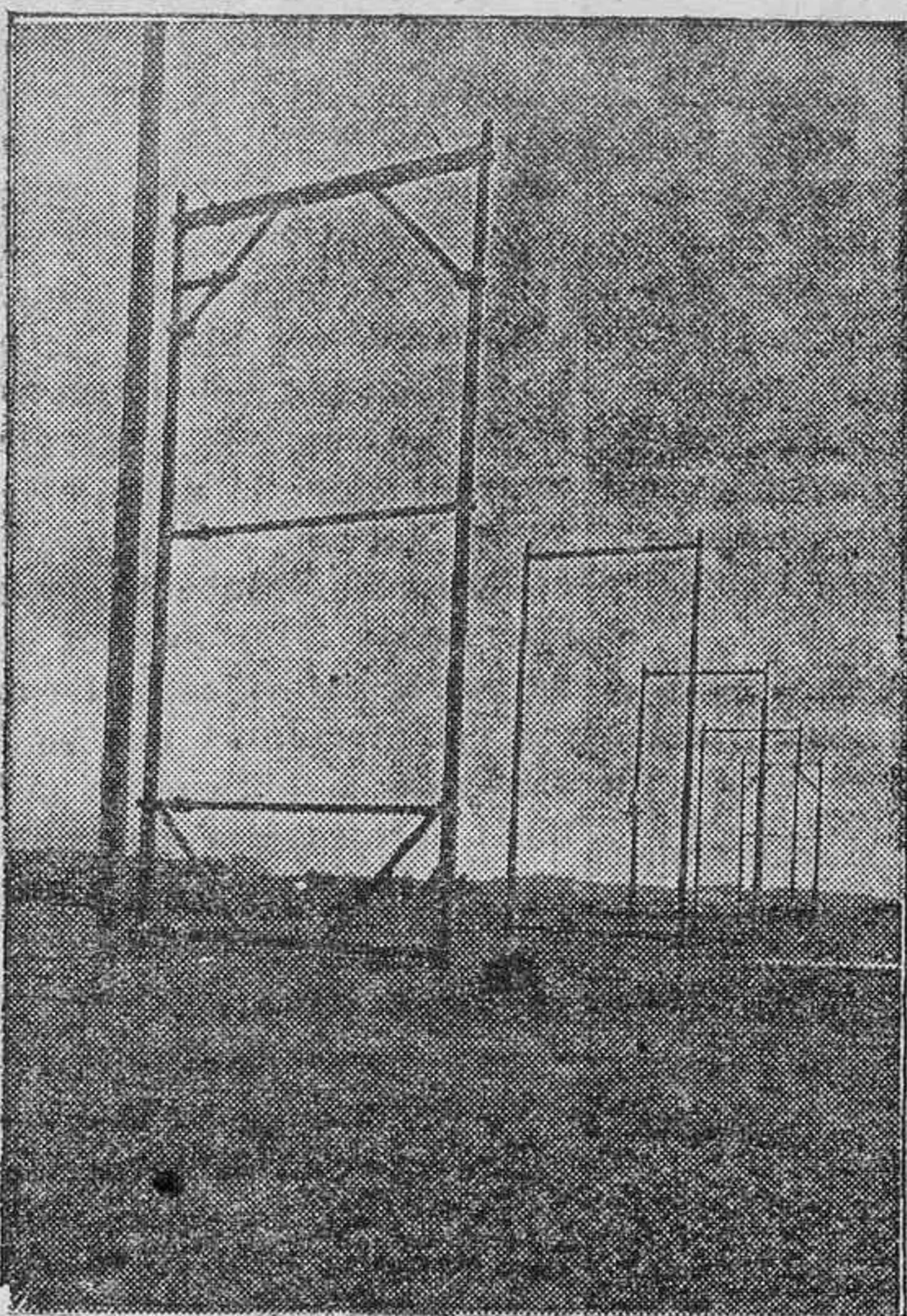
EL TELEFONO CON LA PENINSULA.—Dos detalles de la Estación de El Tablero. Grupo de antenas receptoras. Equipo receptor y de control de radio.—(Fotos Benítez).
