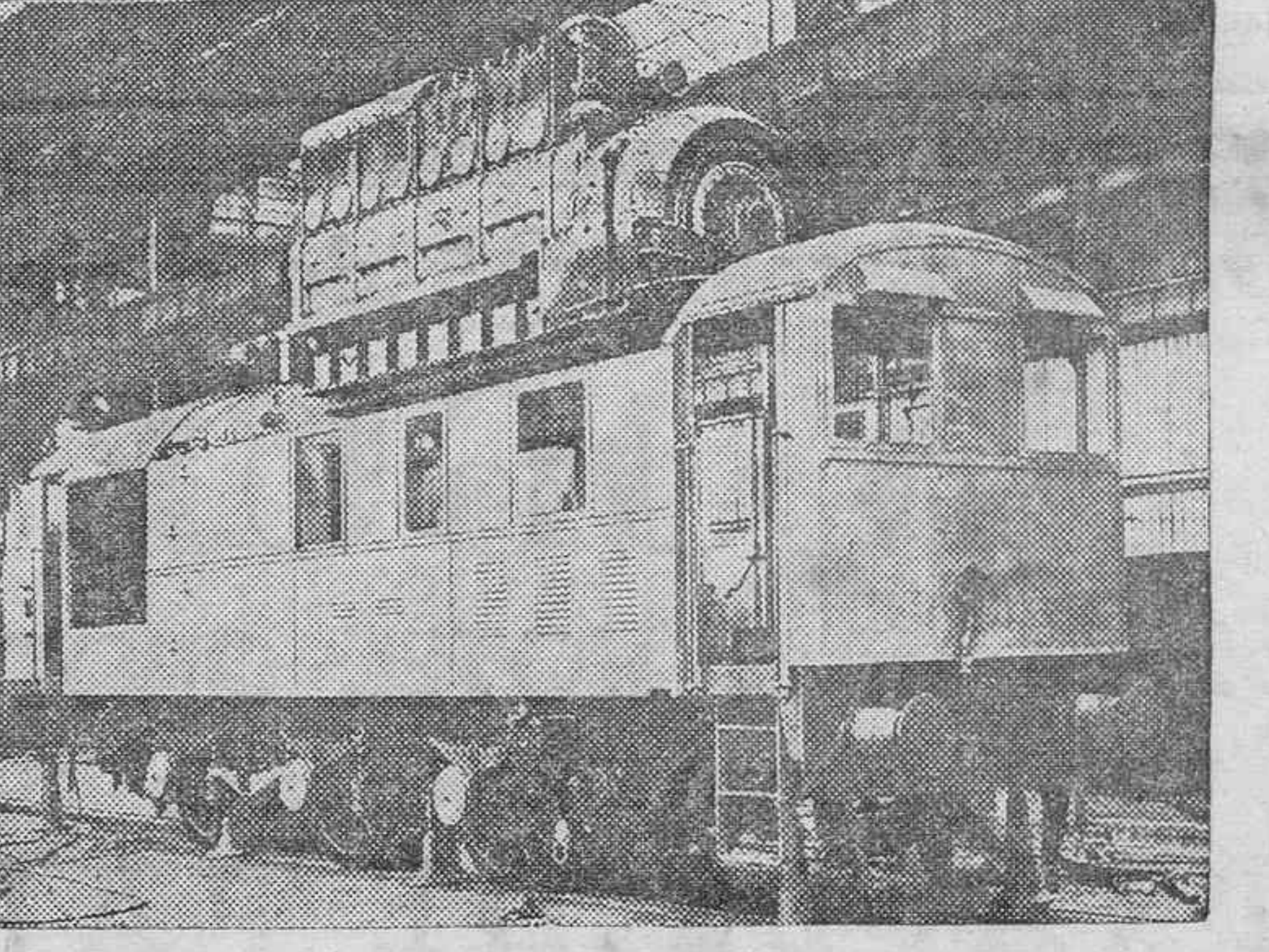
EL NUEVO TIPO DE LOCOMOTORA INGLESA. TRATASE DE UNA MAQUINA DIESEL, QUE SE EMPLEA PARA LOS FERROCARRILES, OMNIBUS Y HASTA TRENES EXPRESOS.
