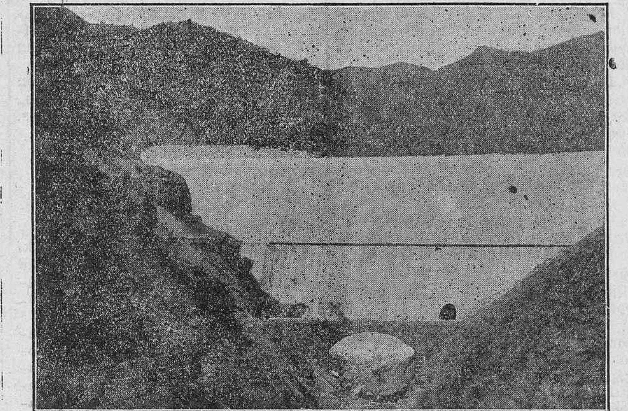
VISTA EXTERIOR DEL MURO DE PRESA, CUYO ALTO ACTUAL ES DE 26 Y MEDIO METROS
