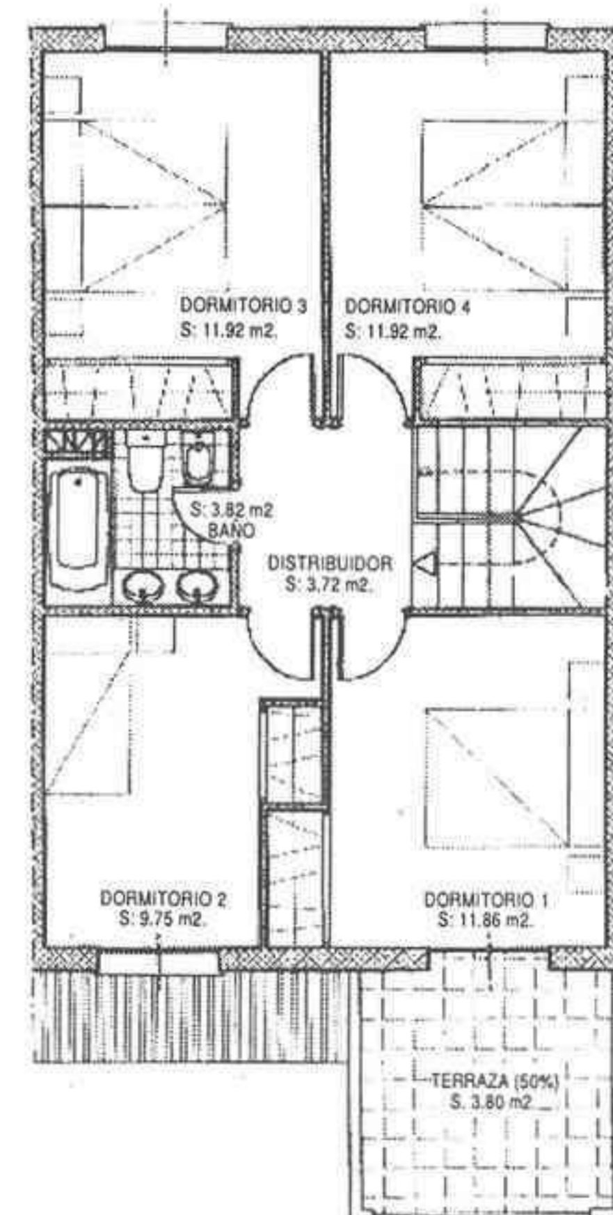
PLANTA ALTA
