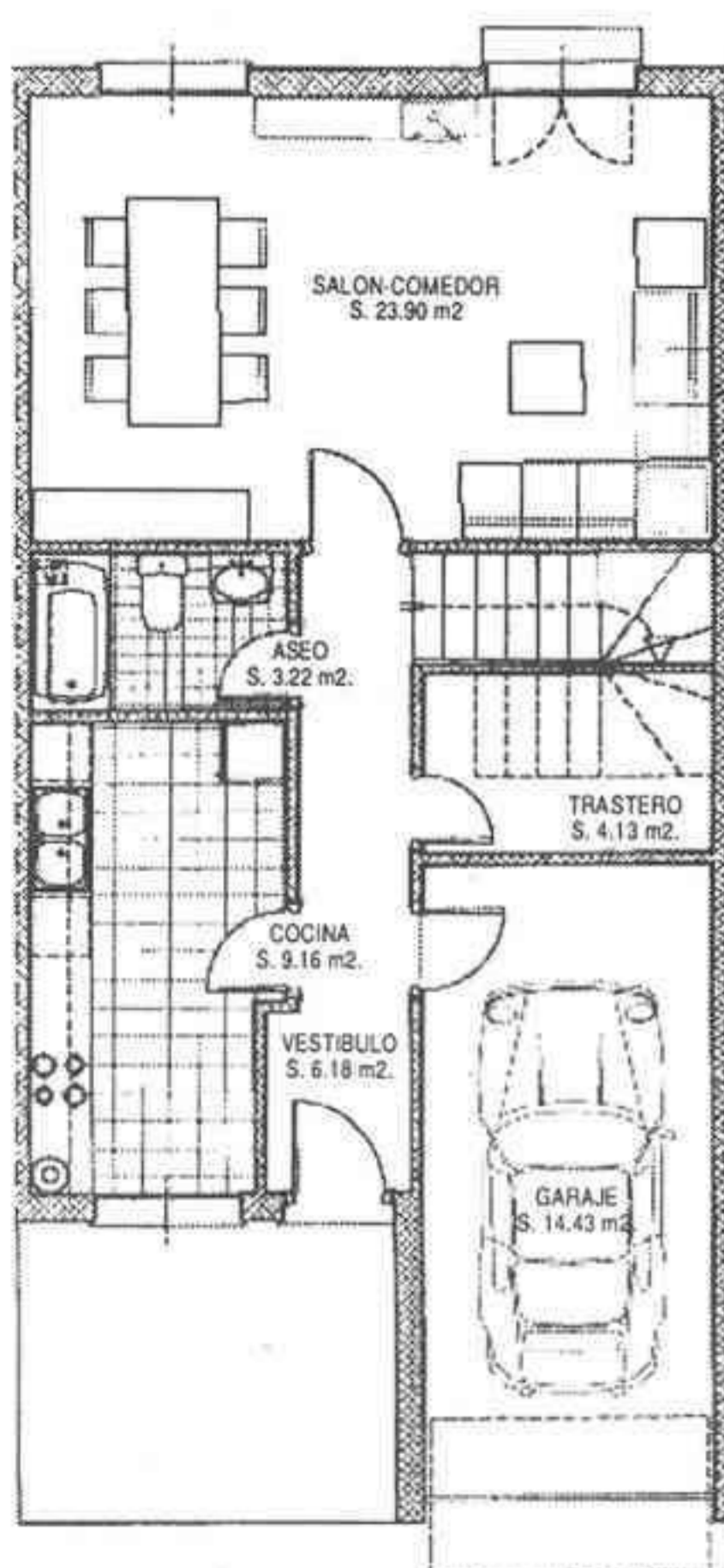
PLANTA BAJA
