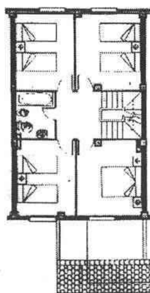
PLANTA PRIMERA
