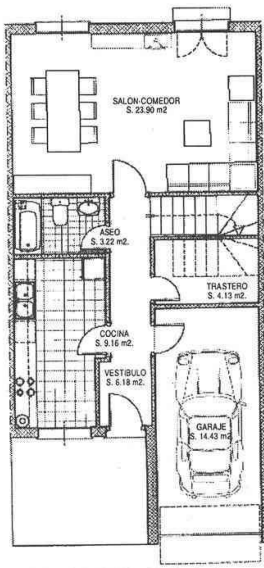
PLANTA BAJA
