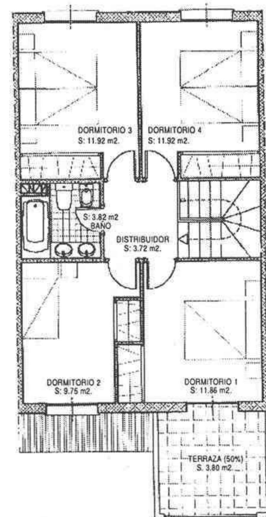
PLANTA ALTA
