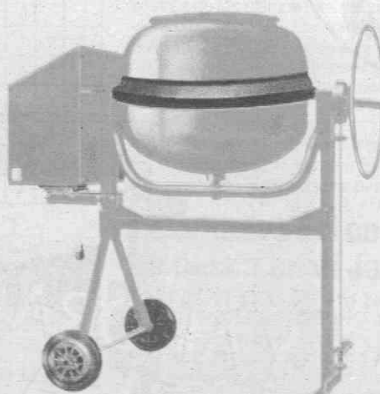
Hormigonera MB-120 MOM Cuba 120 litros. Peso 65 kg Potencia motor 0,4 CV
