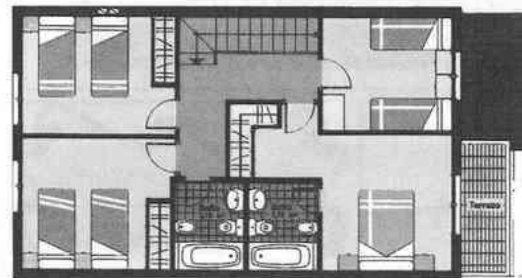
Planta PRIMERA
