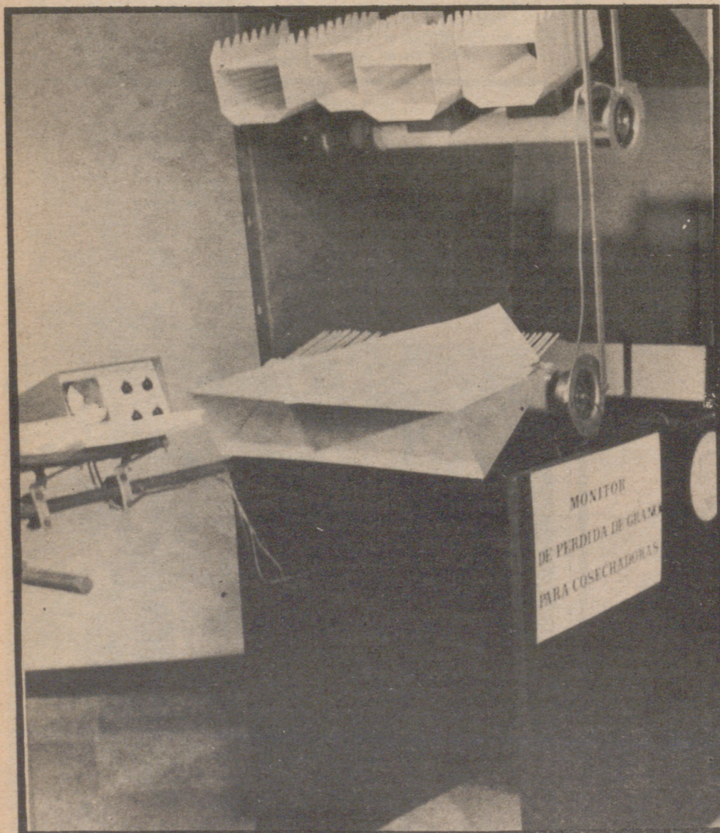
Este es el magnífico aparato monitor de pérdida de grano para cosechadoras. Su efectividad es completa y las garantías totales.
