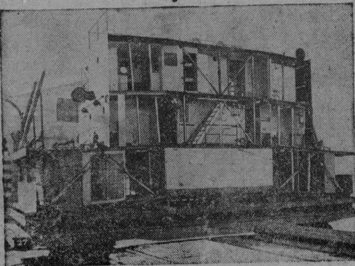
Una sección del "Robert E. Feary" transportada sobre un remolque para ser instalada en el barco. Este buque fué botado a los 4 días y 15 horas y media de haberle puesto la quilla.
