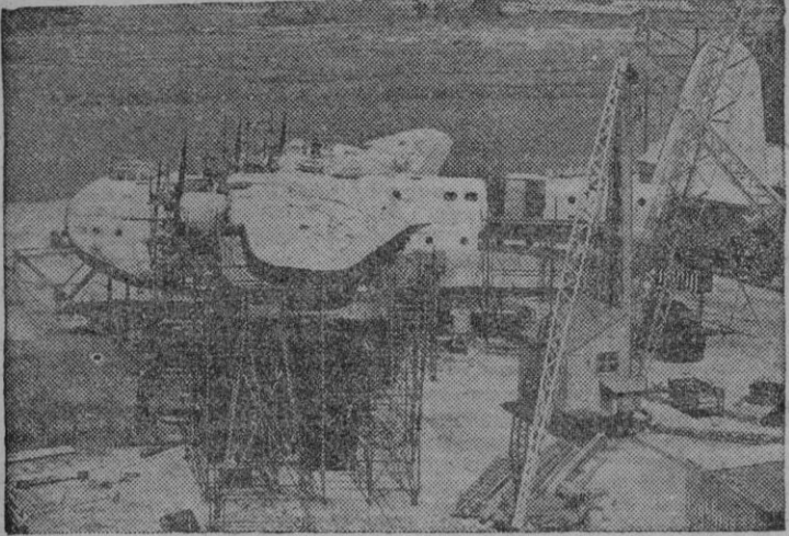
El gigantesco avión británico «Short-Saro Shetland» en las gradas a orillas del río Midway. Como se vé, la construcción de un avión de ese tipo no difiere de la de un trasatlántico.
