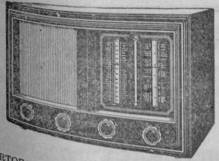
VERTOR modelo W4D, 5 lámparas de funciones completas de 8 dial vertical de plena visión. No obstante su precio económico captó todo el mundo y la calidad de sus componentes hacen del mismo un receptor para muchísimos años. Provisto de antifading. Precio v. p. 1.760 pesetas (i. l.)
