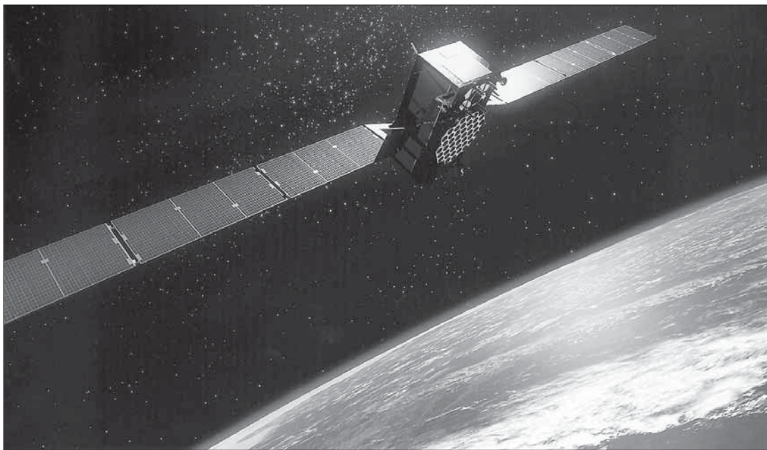
Imagen simulada de un satélite del tipo Galileo en su órbita a través de la Tierra. / EFE
