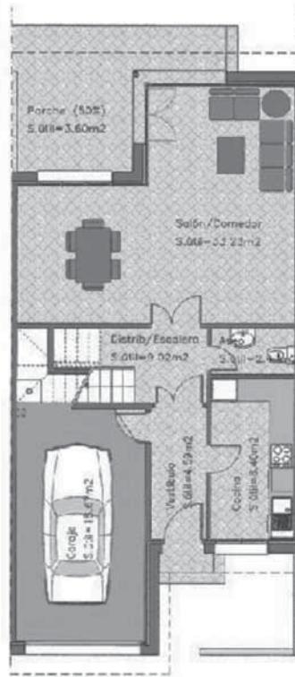
Planta baja S.const.=93,08m 2
