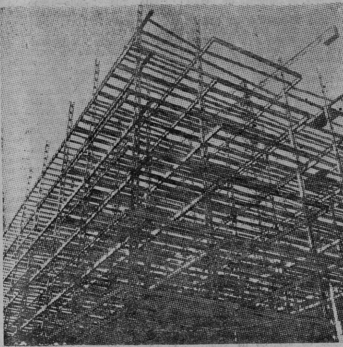
Una vista de la imponente estructura metálica, que ha sido visitada hoy por los alumnos de la Escuela Politécnica del Ejército. La longitud total de las viguetas utilizadas es de 160 kilómetros. (Foto Numay.)
