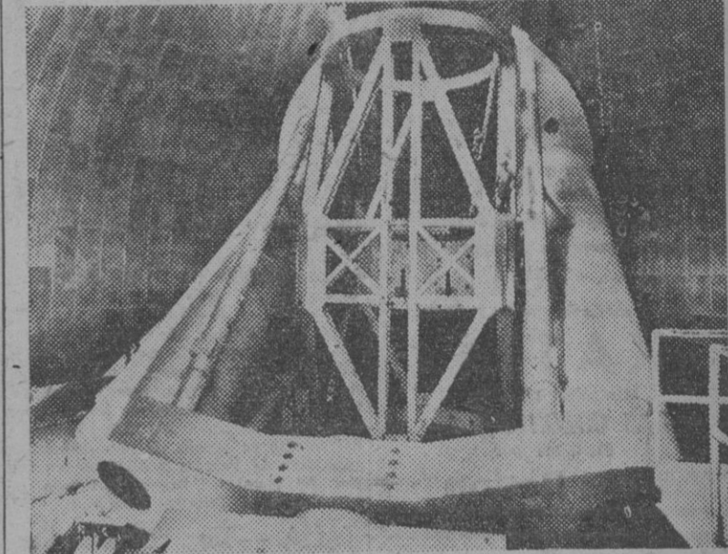
He aquí un aspecto del gigantesco telescopio que se construye para ser instalado en el Monte Palomar (California), donde está situado el Observatorio a que hace referencia este reportaje.
