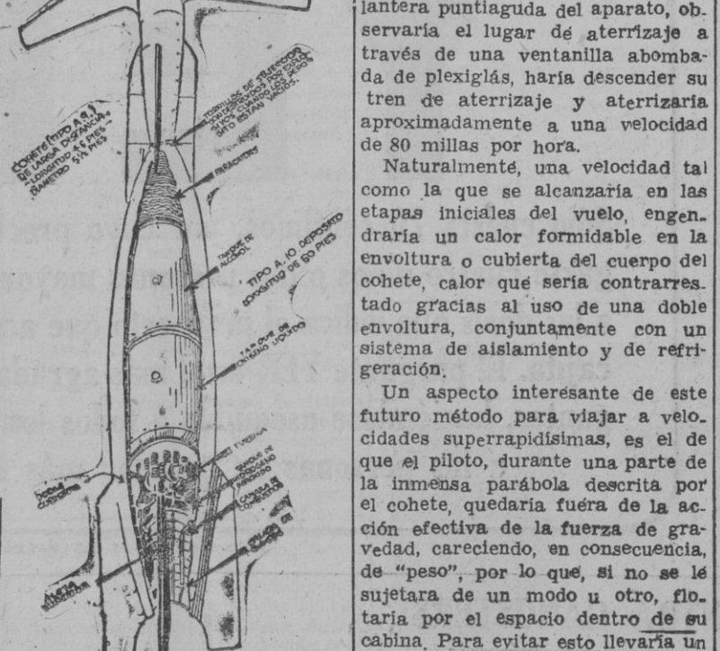
"Aparato auxiliar de impulsión de tipo A 10; longitud, 60 pies, diámetro del cuerpo, 11 pies"
