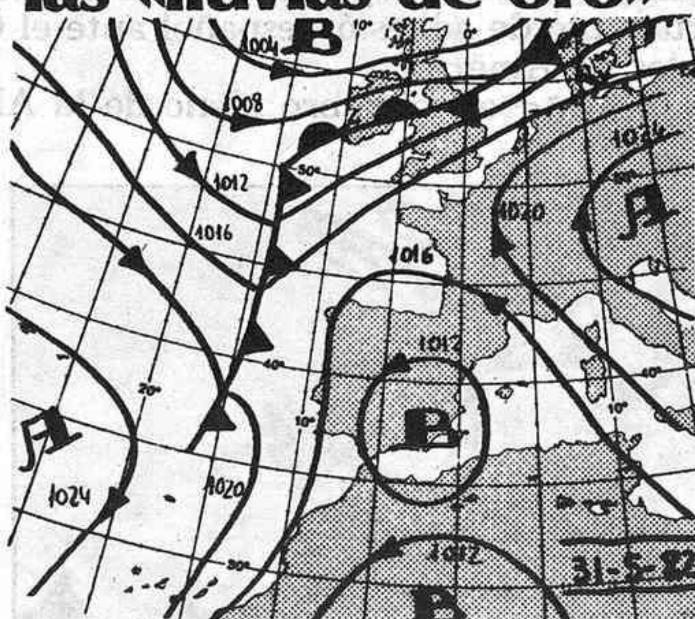
Inestabilidad atmosférica en las capas altas de la atmósfera sobre la vertical del centro peninsular
