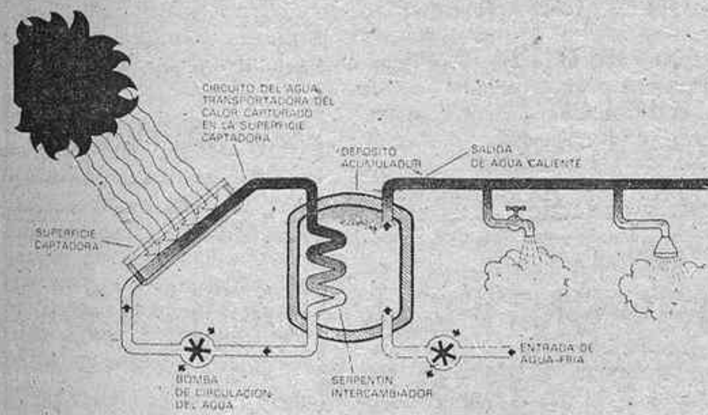
Esquema de un sistema de captación de energía solar para el suministro de agua caliente
