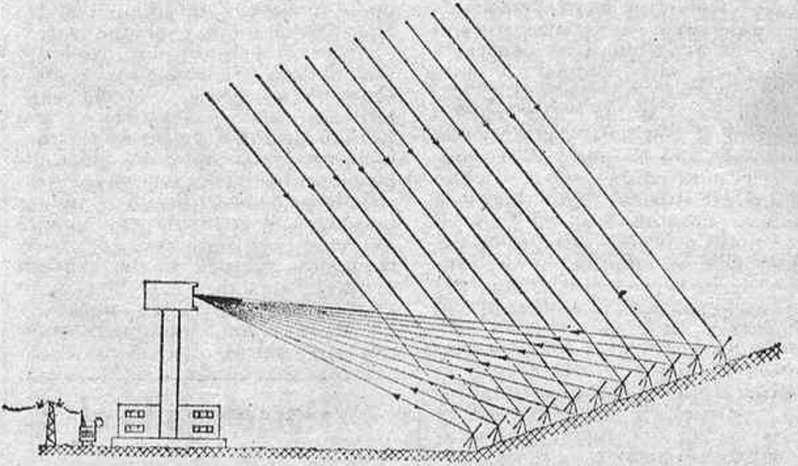
El gráfico representa cómo los espejos reflejan los rayos solares que inciden sobre ellos, enviándolos a un receptor montado en la parte superior de la torre
