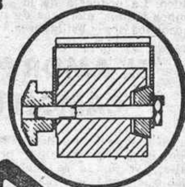
dispositivo de freno de las ruedas delanteras
