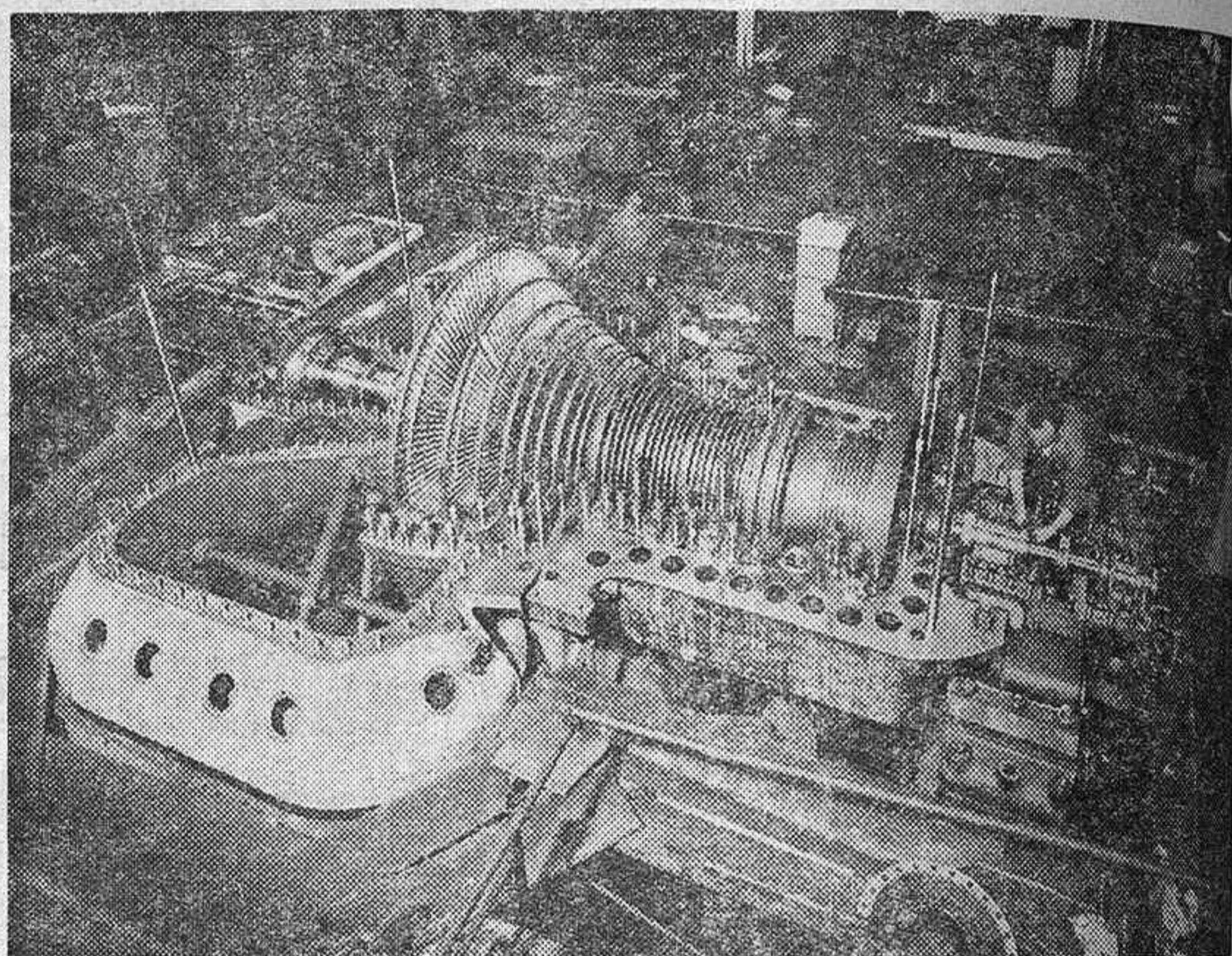
Turbina de 40 M. W. Medición de huelgos entre rotor y base cilindro.
