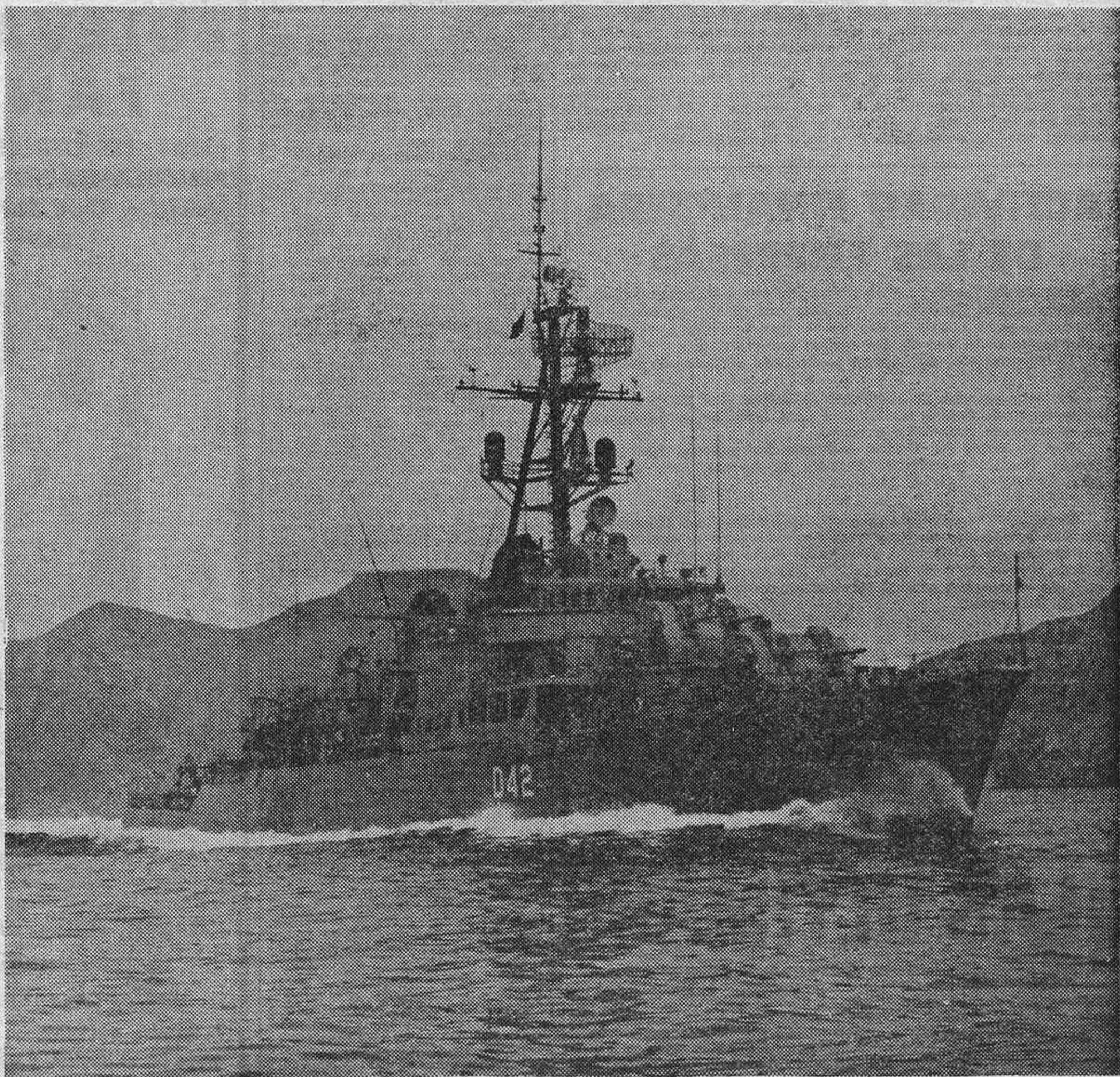
Destructor "Roger de Lauria" para la Marina de Guerra española.
