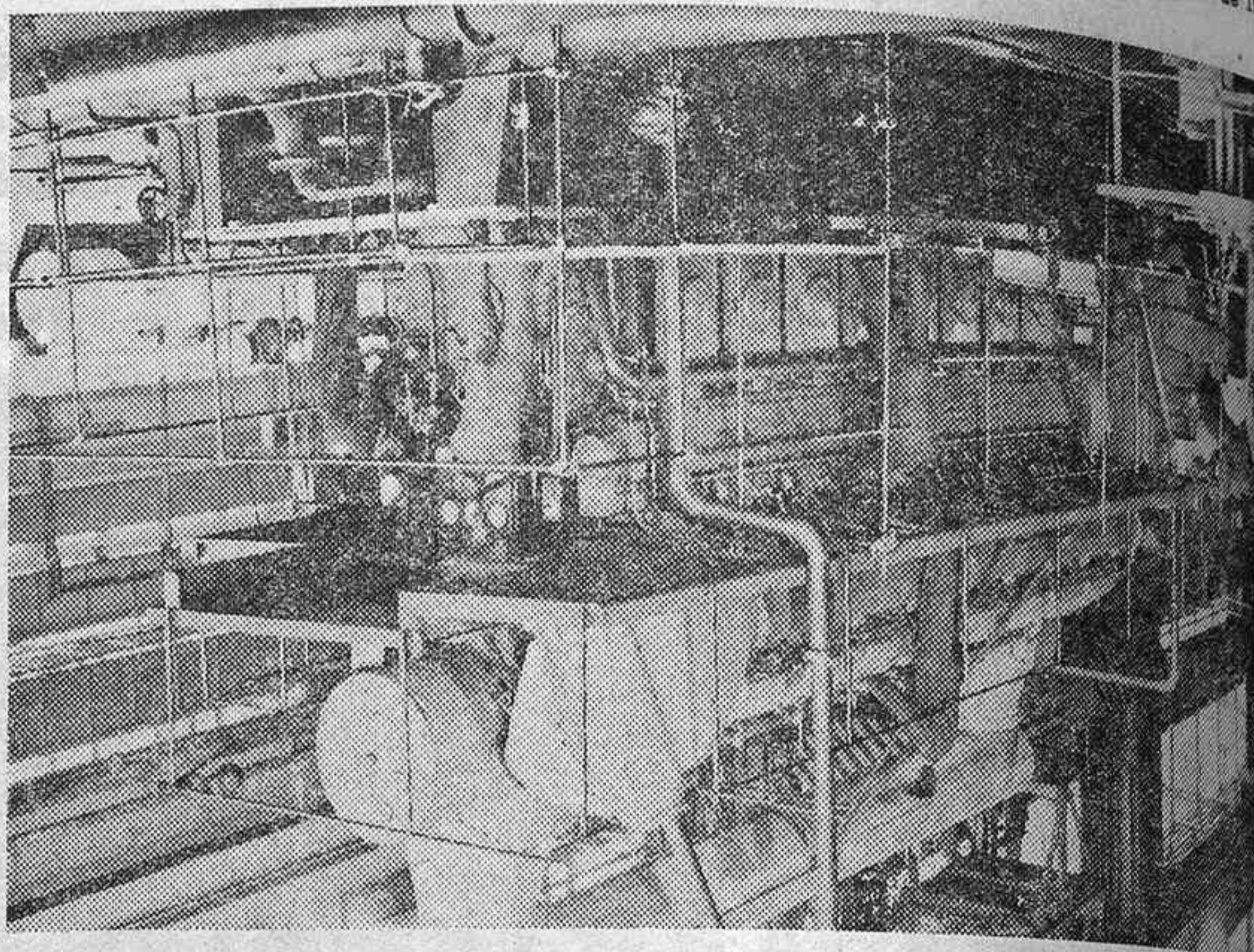
Motor Bazán-Man tipo 40/54.
