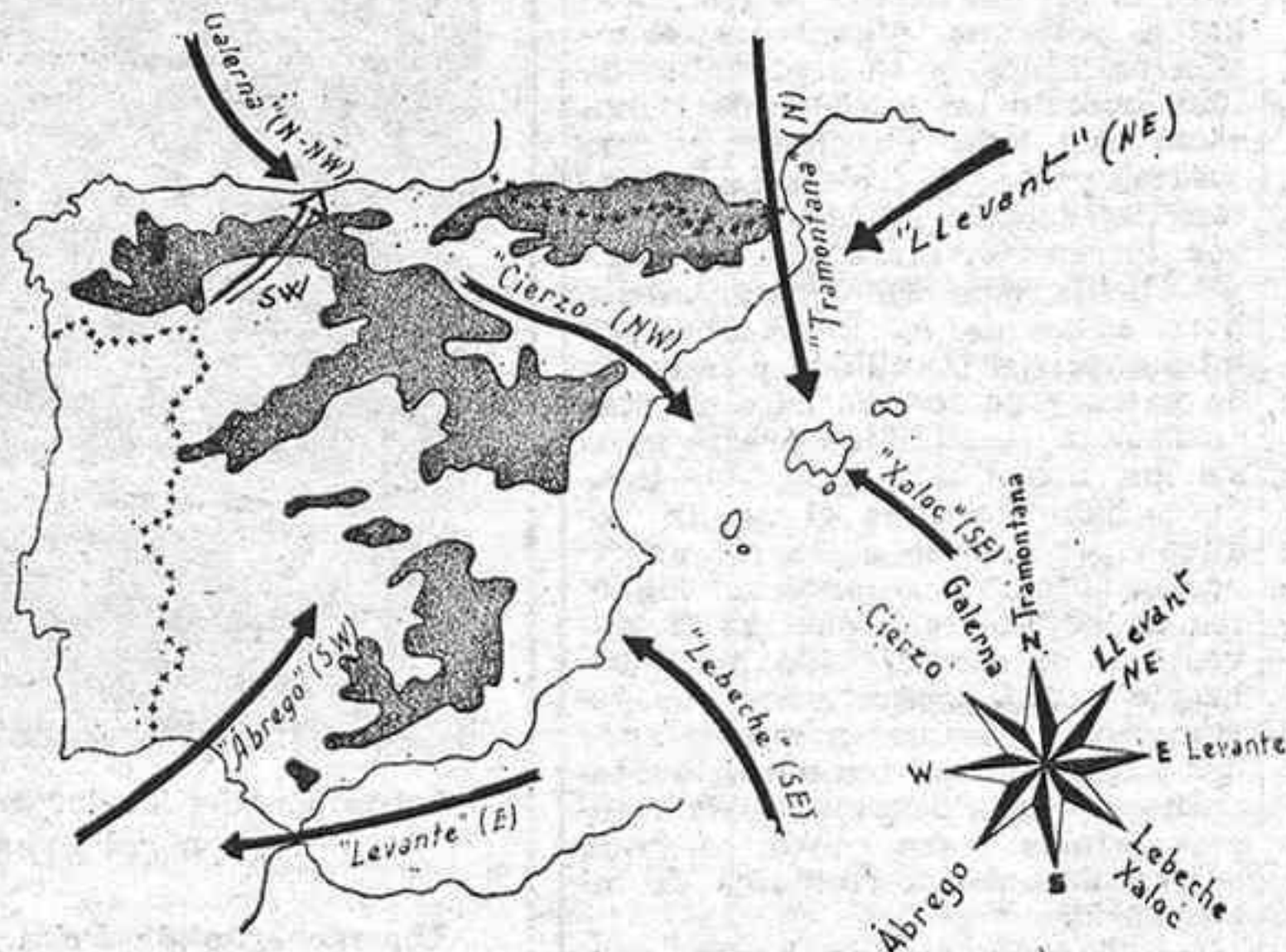
Vientos típicos en España. (Mapa original del autor.)
