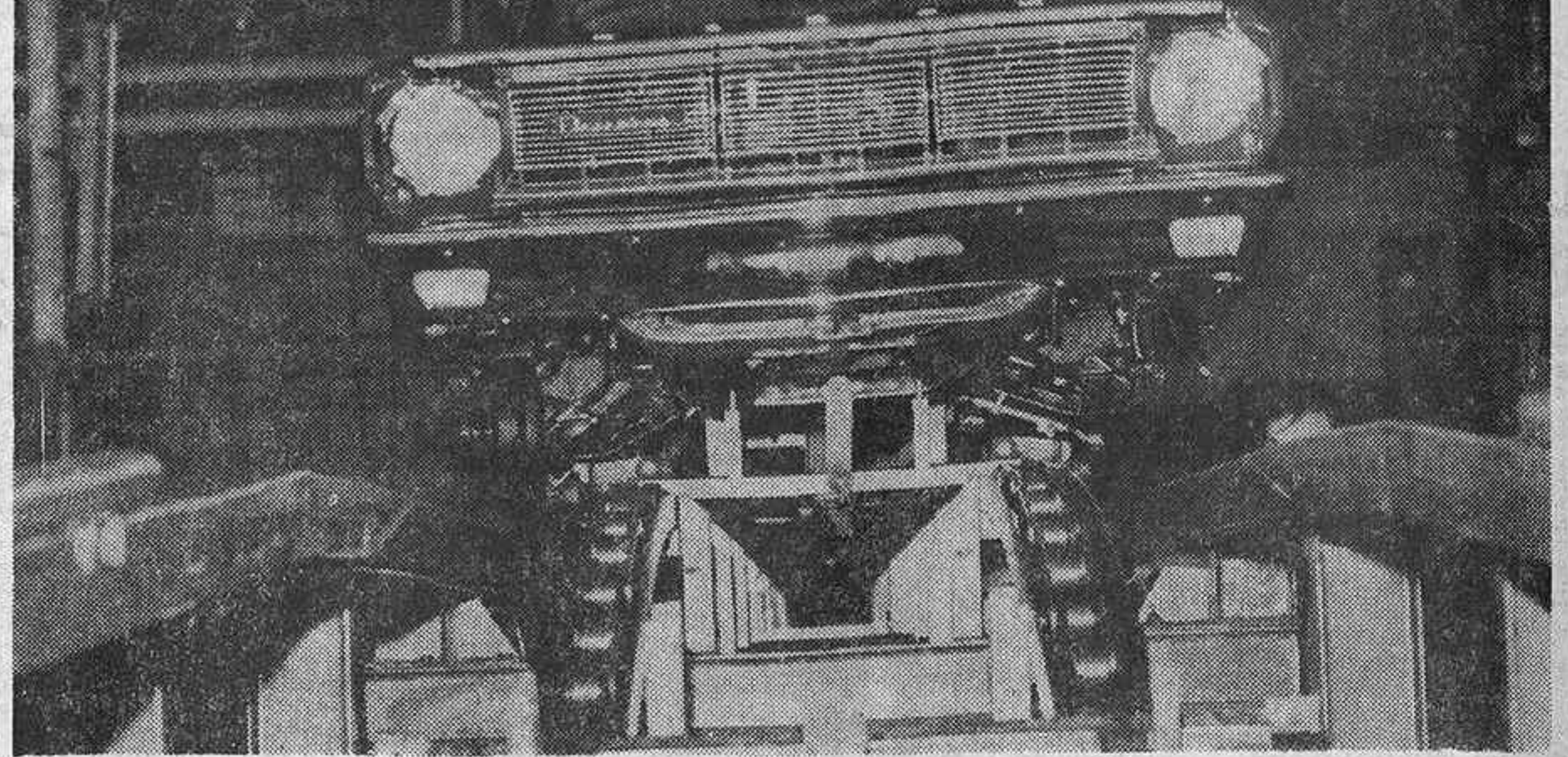
En las cadenas móviles de fabricación, el Dodge va recibiendo los distintos elementos mecánicos, en su mayoría ya nacionalizados
