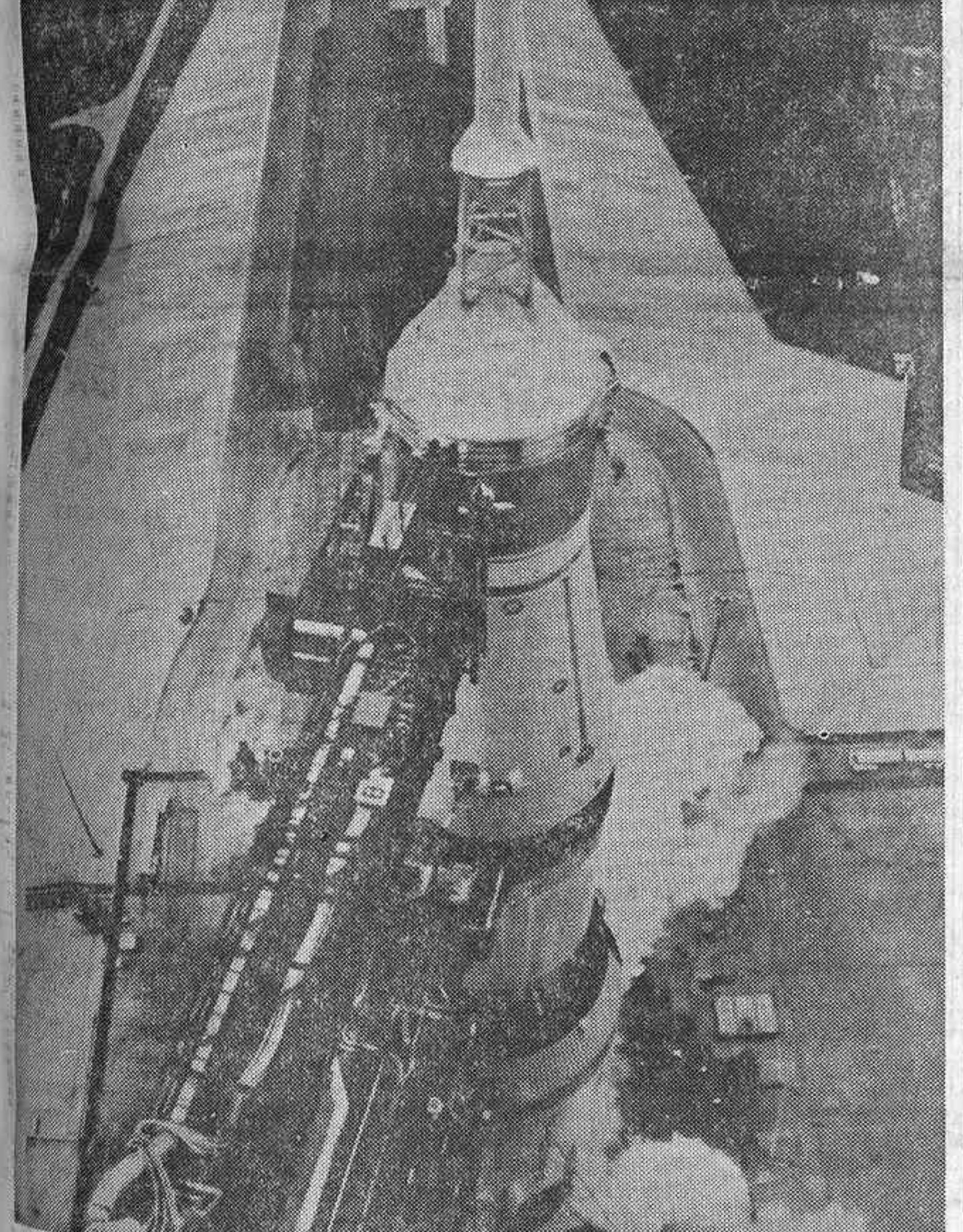
El "Saturno 5", que llevará al "Apolo 11" a la Luna, aparece en pruebas de oxígeno cuando la ya famosa cuenta atrás ha comenzado. (Telefoto Upi-Cifra.)
