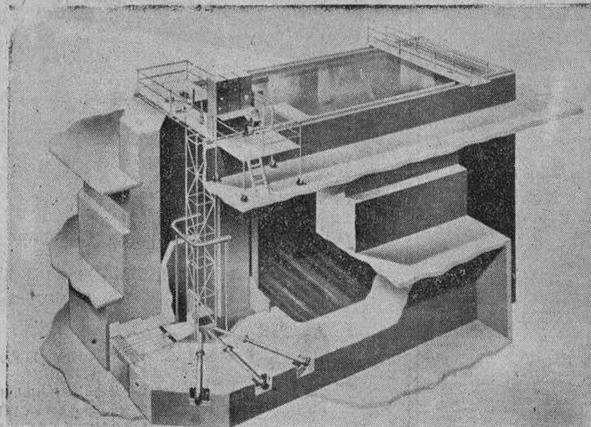
Esta sección vertical del reactor de 3.000 kilovatios de capacidad térmica que será instalado en terrenos de la Moncloa, de Madrid, muestra su disposición interior. El primer reactor de este tipo fue construido en 1951, y en 1955, los delegados de España y de otros 80 países pudieron verlo expuesto en Ginebra durante la conferencia de "Átomos para la paz". La seguridad y las múltiples posibilidades de este tipo de reactor hacen que sea ideal para investigaciones científicas.
