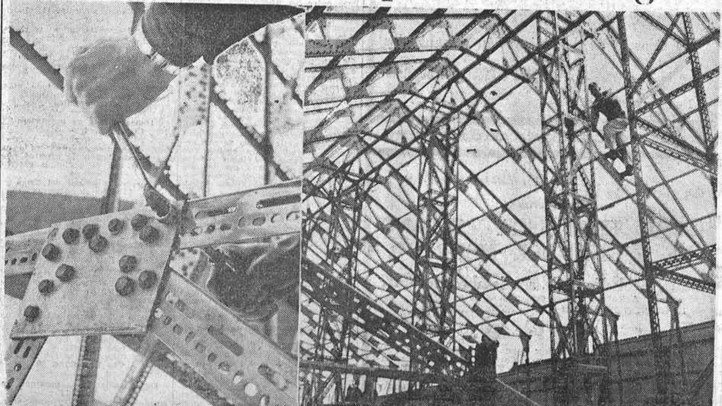
Las modernas estructuras metálicas para fabricación de grandes naves y otro género de edificios, como muestra la foto de la derecha, apenas si exigen otro instrumental que la llave inglesa para apretar las tuercas, como se demuestra en la izquierda. Corresponden ambas a una fábrica de Copenhague. El sistema no puede ser más rápido y sencillo. (Foto Torremochá.)
