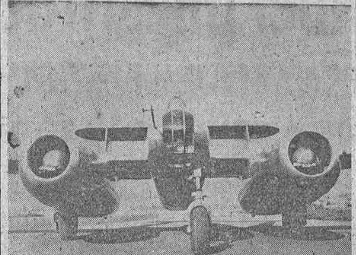
El aparato que reproduce la fotografía es el primer avión bimotor de reacción fabricado en Francia. Es el N. C. 1071, tiene 20 metros de envergadura y 10 de longitud y desarrolla una velocidad de 700 a 800 kilómetros por hora. Su autonomía de vuelo es de 8.000 metros. (Foto Cifra).
