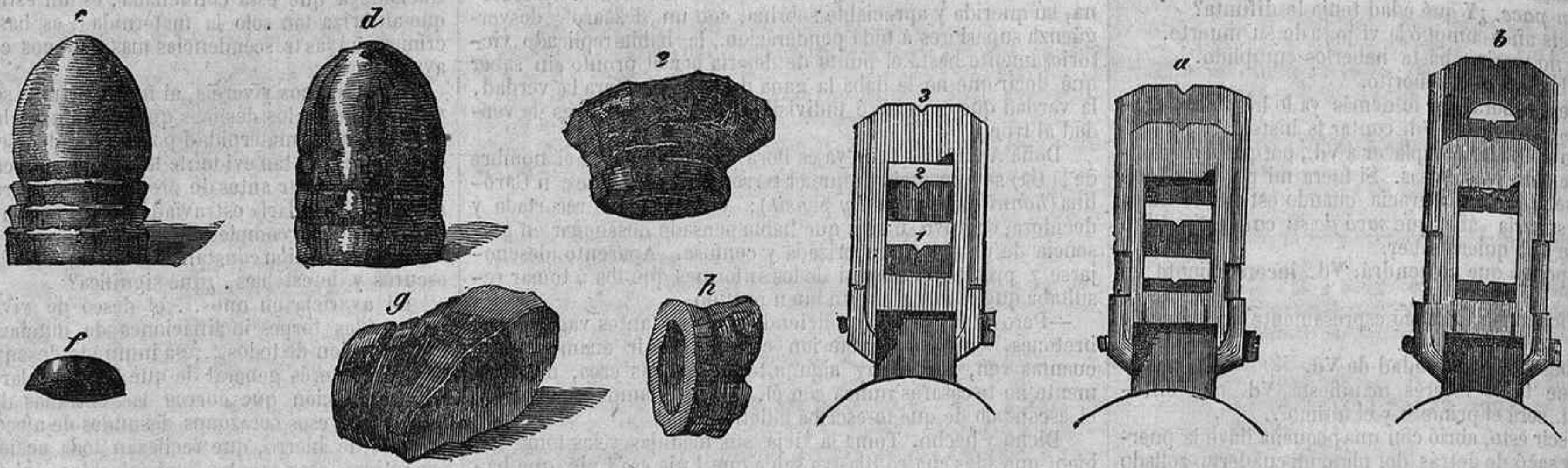
DETALLES DEL FUSIL DE MINIÉ.—a Puente de mira para 900 pasos de distancia.—b Puente de mira para 1,000 pasos de distancia.—1 Mira de 2/3 de su dimension natural para 400 pasos de distancia.—2 Mira de 2/3 de su tamaño natural para 600 pasos de distancia.—3 Mira de 2/3 de su dimension natural para 800 pasos de distancia.—c Bala.—d Bala que disparada no dió contra un objeto duro.—e Bala que fué arrojada contra un cuerpo duro.—f Salero de culote.—g Bala que no tomó su verdadera trayectoria.—h Anilla separada de una bala disparada.
