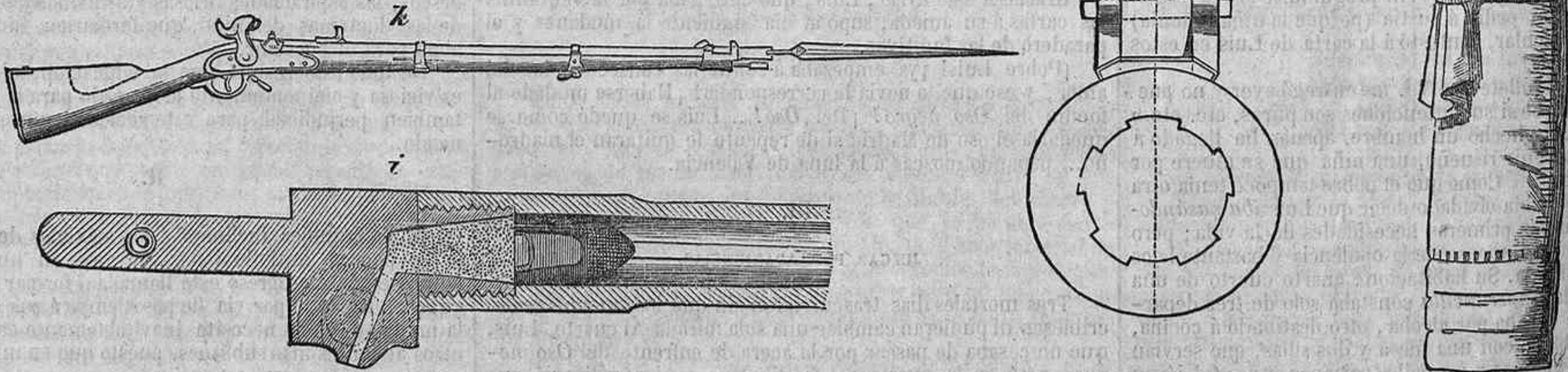
DETALLES DEL FUSIL DE MINIÉ.—4 Mira de dimension natural para 150 pasos de distancia.—5 Mira de tamaño natural para 300 pasos de distancia.—6 Corte trasversal del cañon y de la recámara.—k fusil de Minié.—l Rayas y mira del tamaño natural para 150 y 300 pasos de distancia.—m Cartucho.
