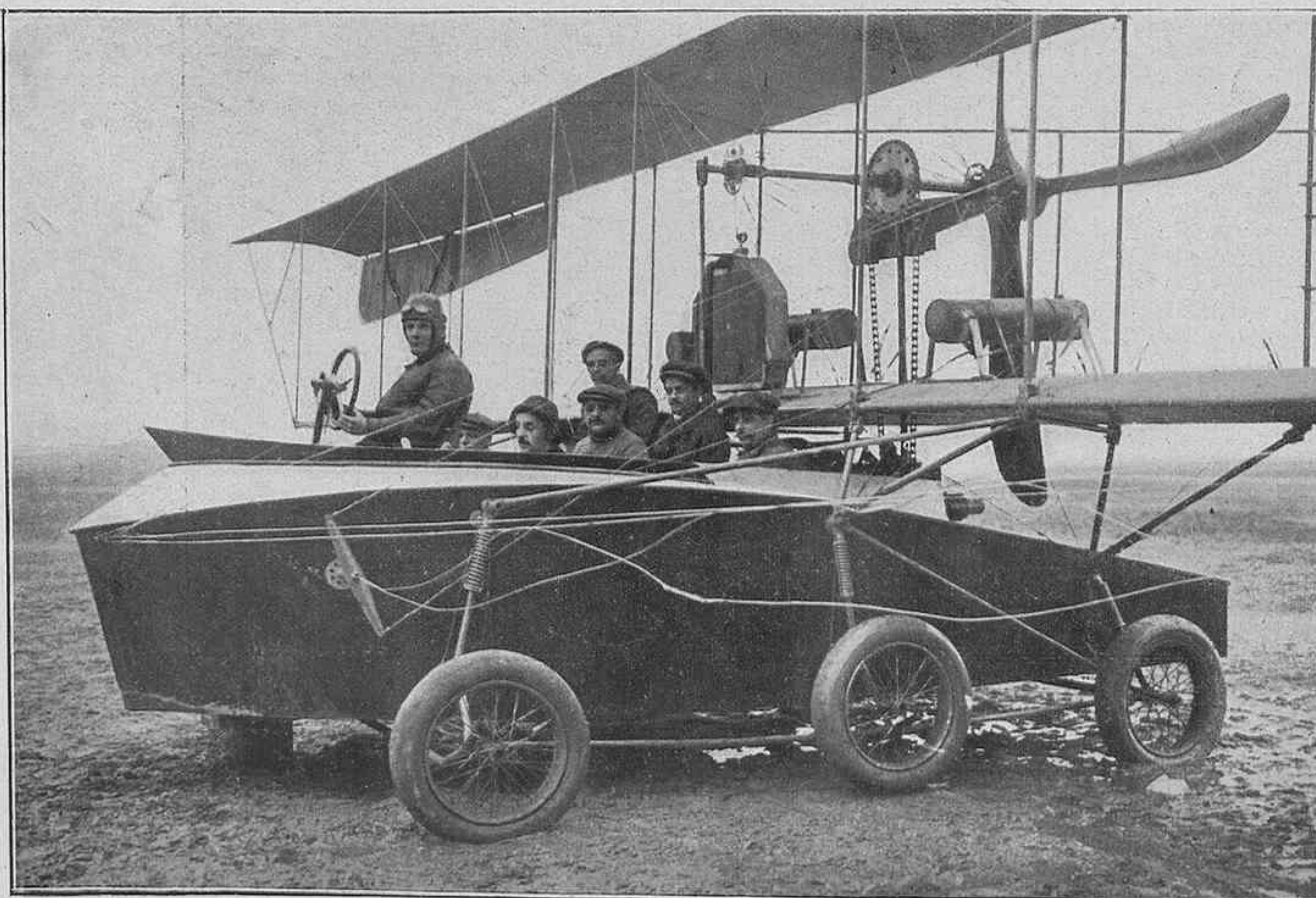
Nuevo hidro-aeroplano construido por Gabriel Voisín, que puede llevar, además del piloto, seis pasajeros y del cual se han hecho recientemente y con éxito satisfactorio ensayos en Issy-les-Moulineaux. (Fot. Rol.)
