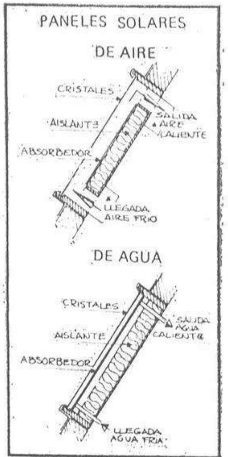
Corte transversal de los paneles solares.
