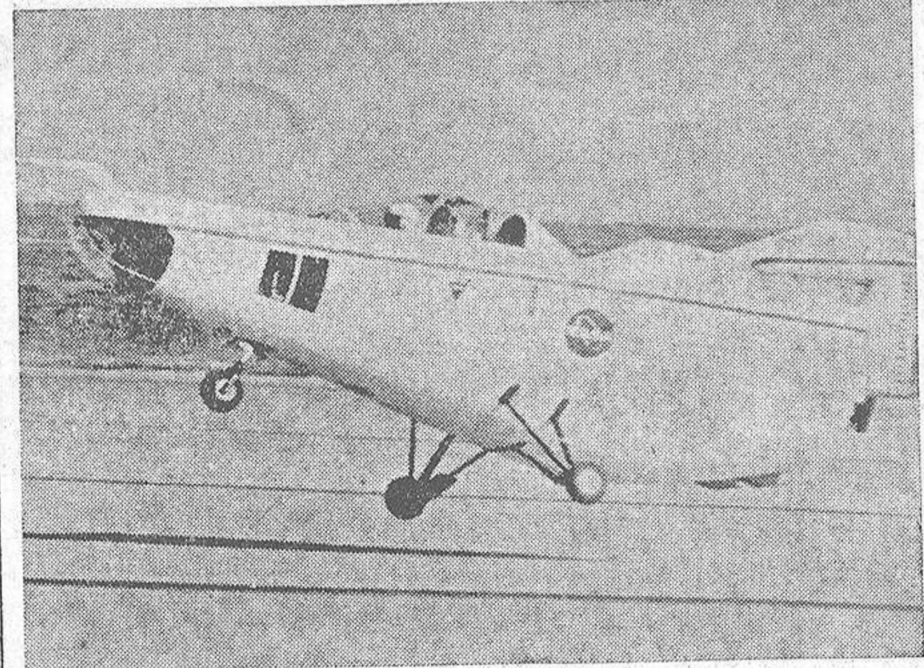
Este es el avión sin alas "M2", en el que el piloto de pruebas de la NASA, Milton O. Thomson experimenta la entrada sin alas en la atmósfera desde una altura de diez mil metros, adonde es izado por un avión "B-52". En principio, este avión está dispuesto para recoger en el aire a los astronautas y puede aterrizar en cualquier aeropuerto comercial. (Foto Efe)
