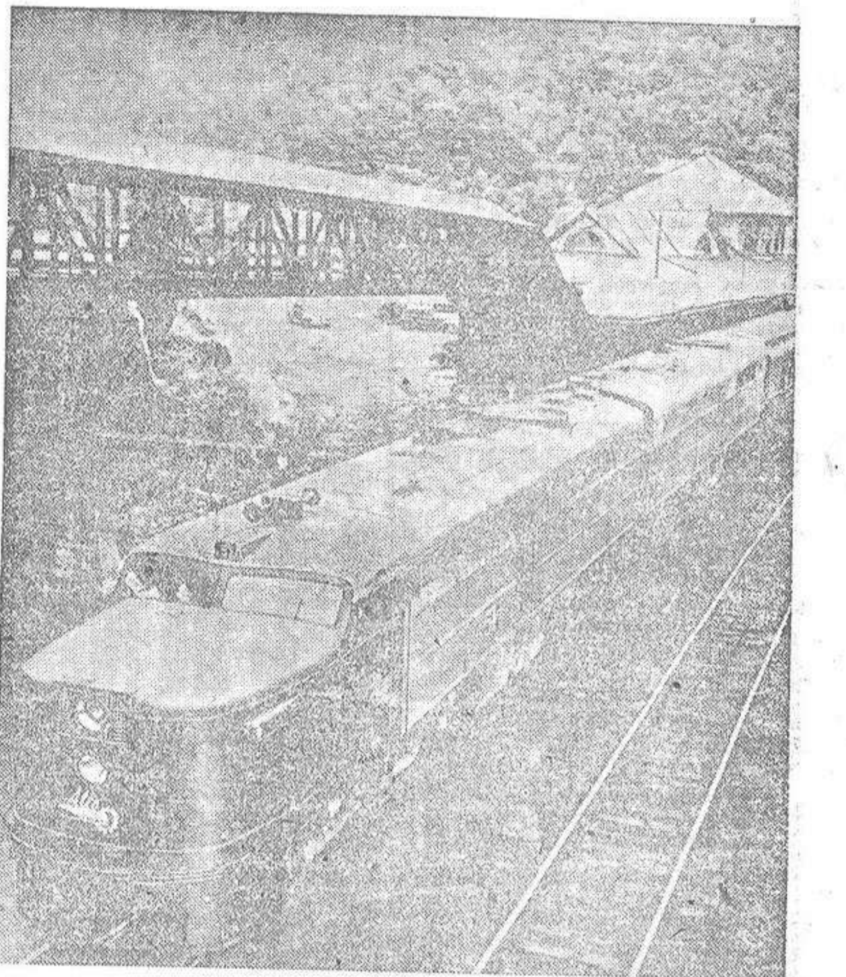
Nuevo tipo de locomotora eléctrica con motor Diesel, de 6.000 H. P., destinada al servicio entre Chicago y varios puntos de la costa del Pacífico. Pesa 450 toneladas y mide cerca de 60 metros de longitud y cuatro y medio de altura. Desarrolla una velocidad de 190 kilómetros por hora. Las pruebas efectuadas en las vías férreas de Pensilvania, dieron un éxito completo.
