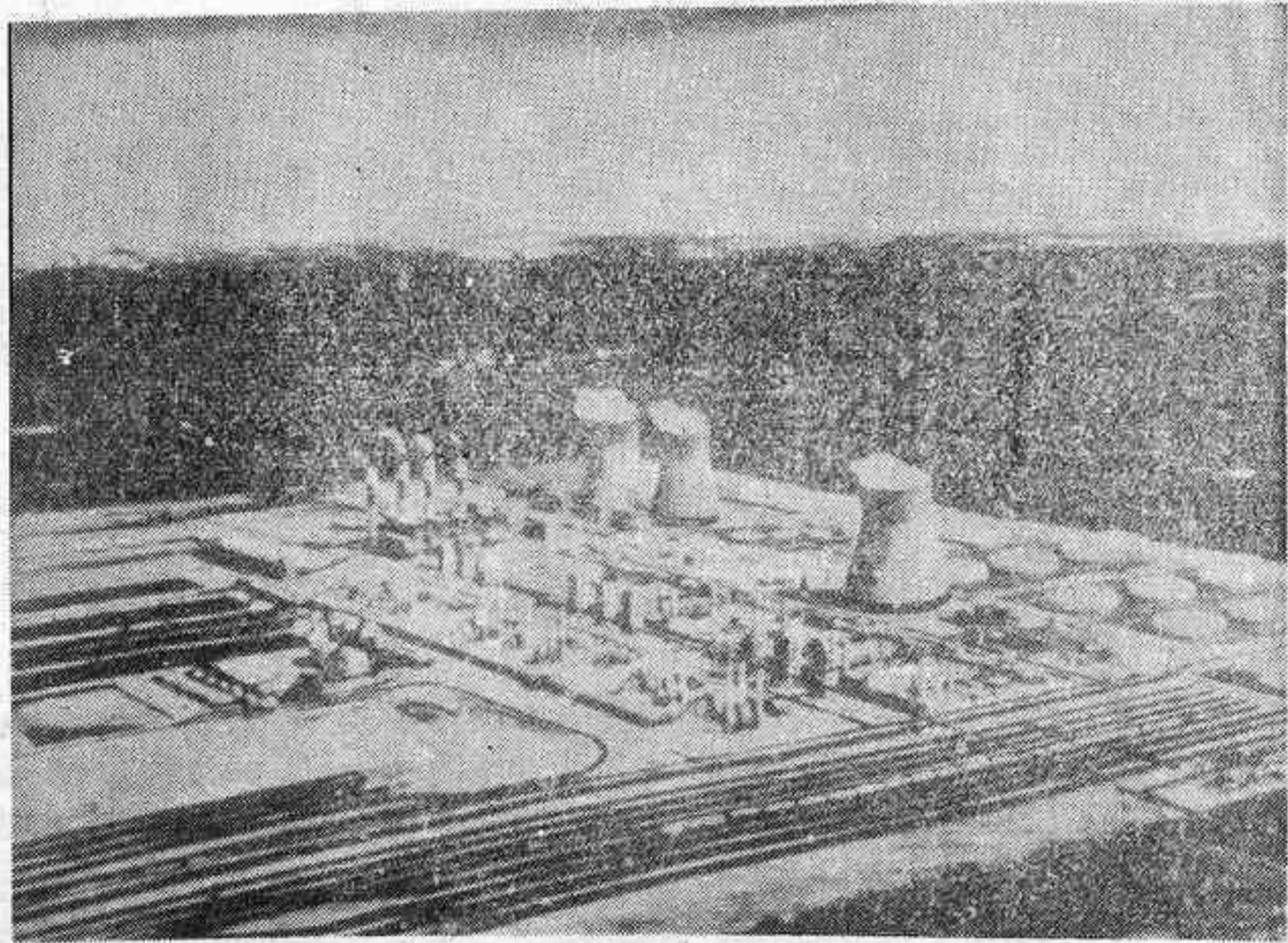
CAMBRIDGE (MASSACHUSETTS). — Dibujo de una planta que podría convertir 63.000 toneladas de carbón en 167.500 barriles de gasolina por día. El diseño se debe a Badger Energy Inc., de Cambridge, y es parte de un estudio para la futura construcción de esta planta, que se edificaría sobre un terreno de 2.300 acres, en enero de 1980. — (Telefoto EFE-UPI).
