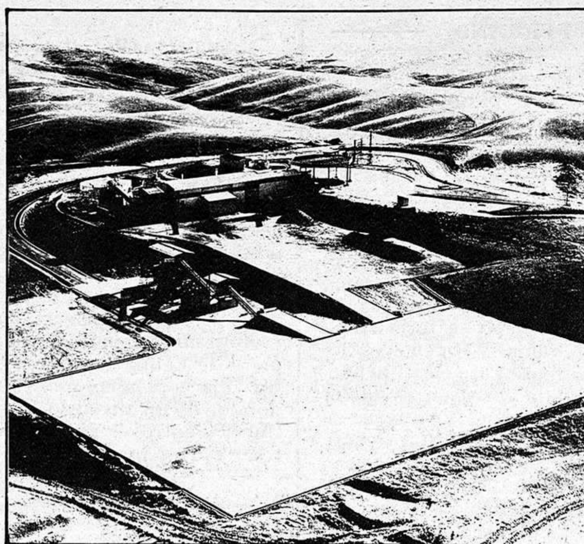
Planta de tratamiento de residuos sólidos (gentileza de Enadimsa)
