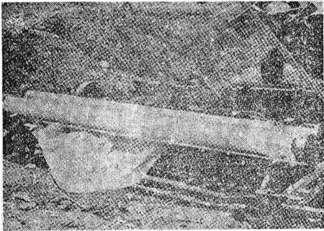
Máquina utilizada para la doble función de sietos, la cual aplica el desinfectante y cubre el terreno con una lámina de polietileno
