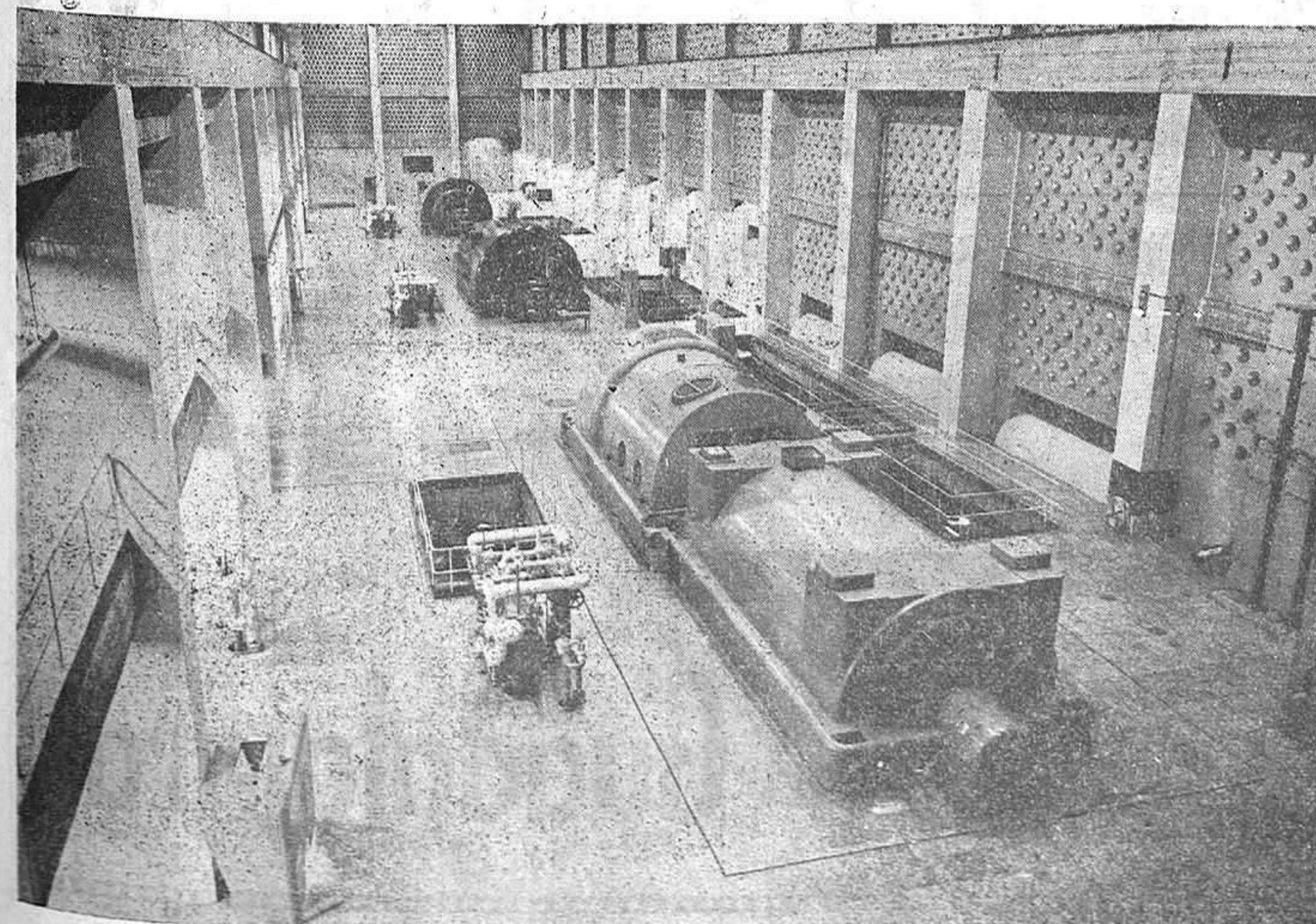
Salto de Alcántara. Potencia: 915.000 kw. Producción anual previsible, 1.800 millones de kwh.
