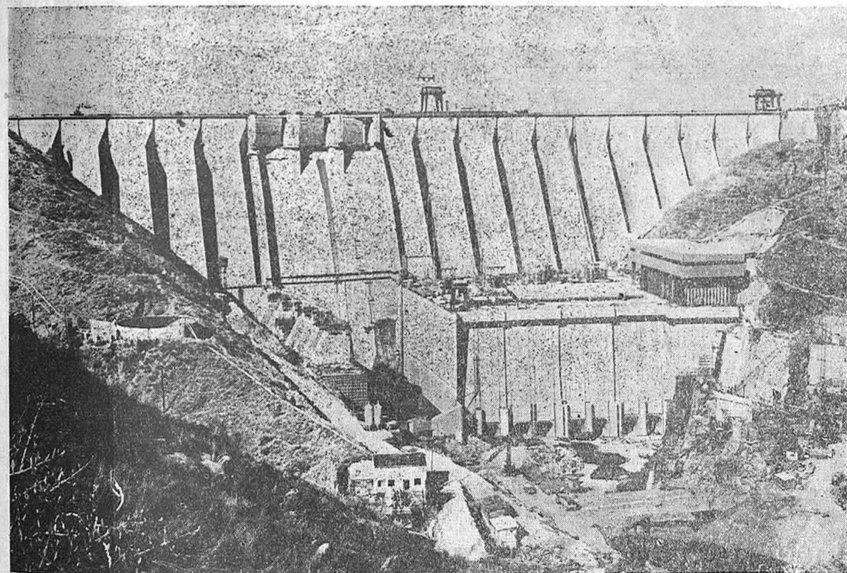
Salto de Alcántara. Potencia: 915.000 kw. Producción anual previsible, 1.800 millones de kwh.
