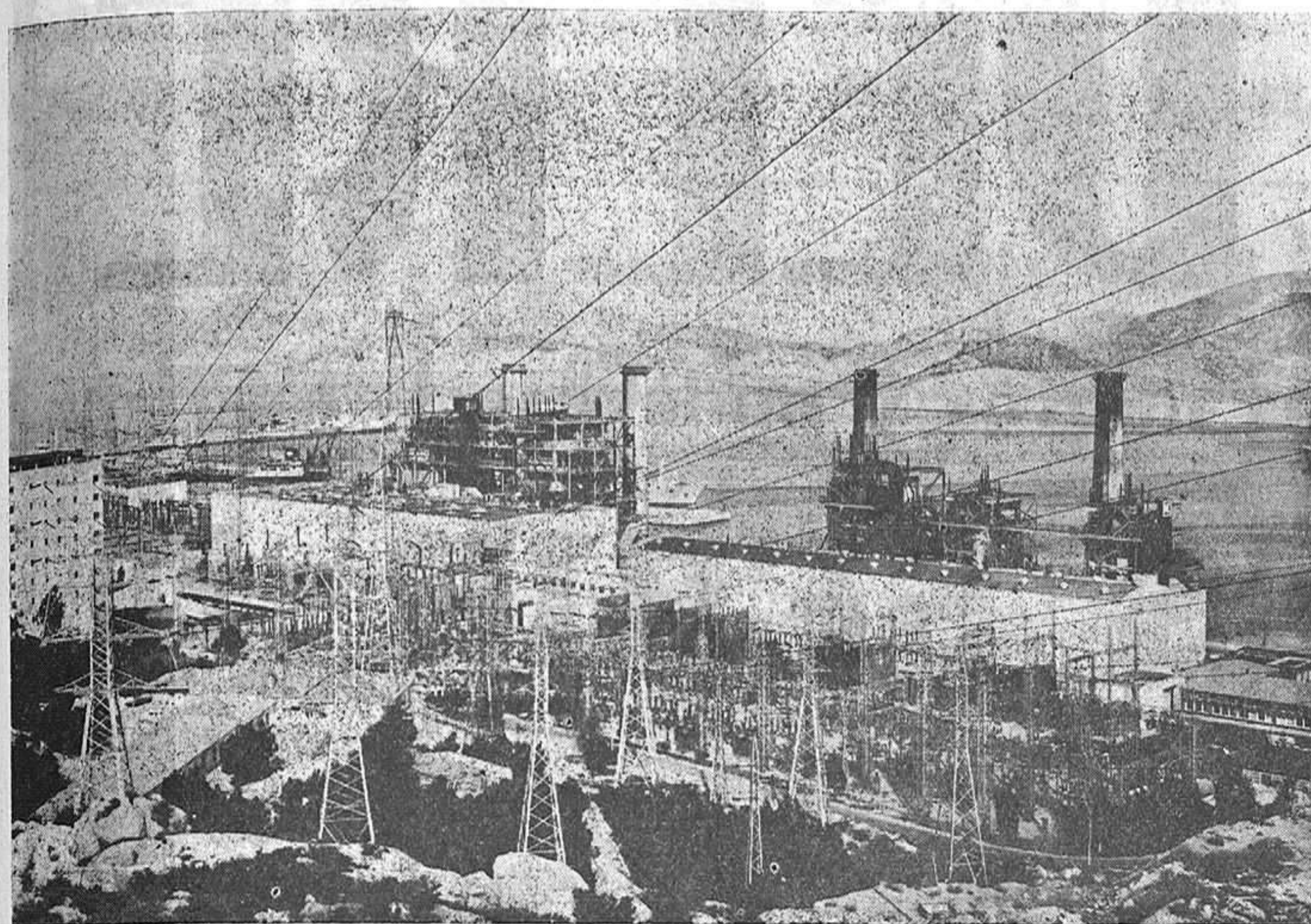
Complejo térmico de Escombreras (Murcia). Potencia: 858.000 kw. Producción anual. 6.500 millones de kwh.
