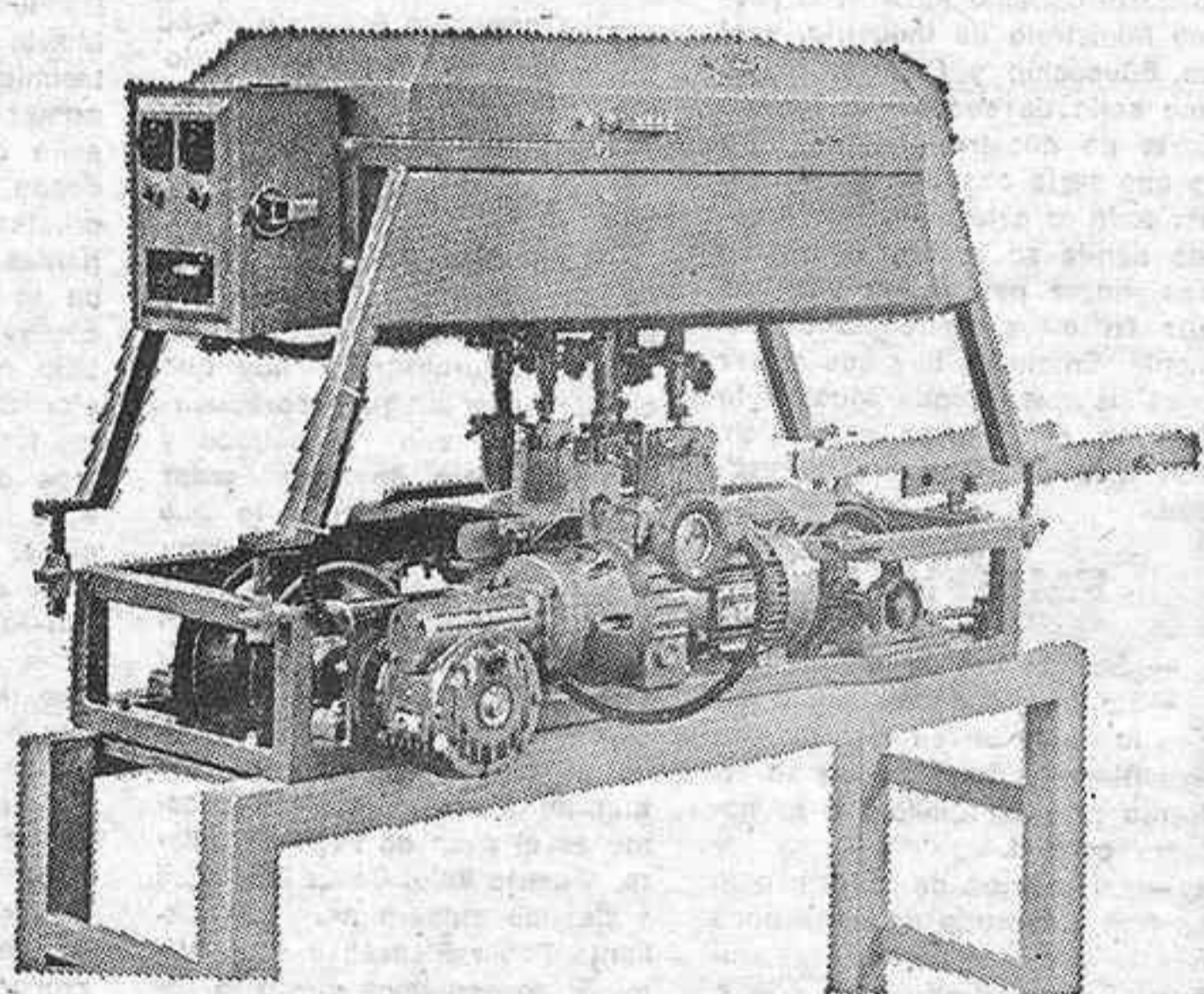
PINCELADORA AUTOMATICA PARA AZULEJOS EN MARCIA CON ESMALTE FRESCO VERTICALMENTE OSCILANTE MODELO 701
