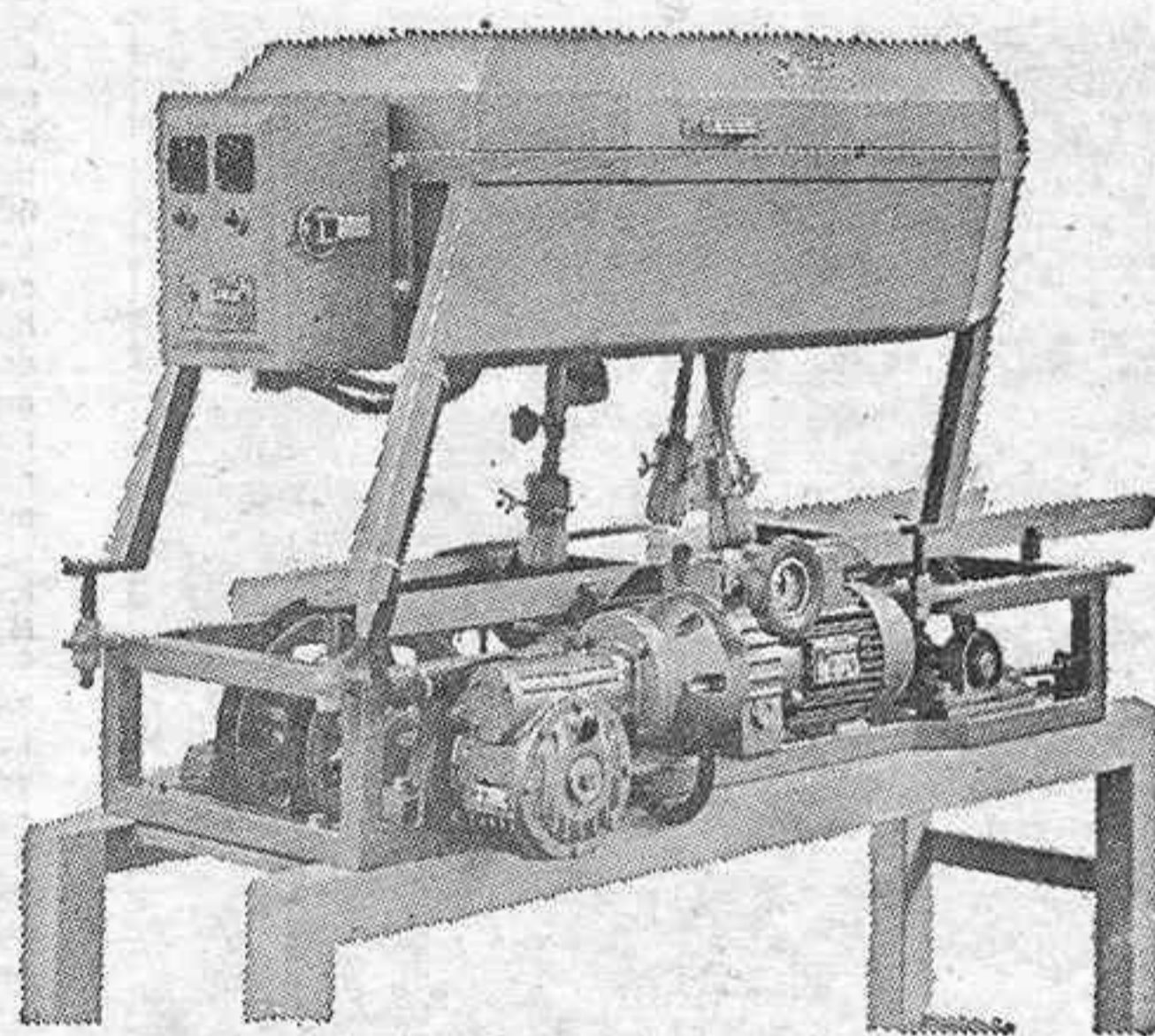
PINCELADORA AUTOMATICA PARA AZULEJOS EN MARCIA CON ESMALTE FRESCO TRANSVERSALMENTE OSCILANTE MODELO 711
